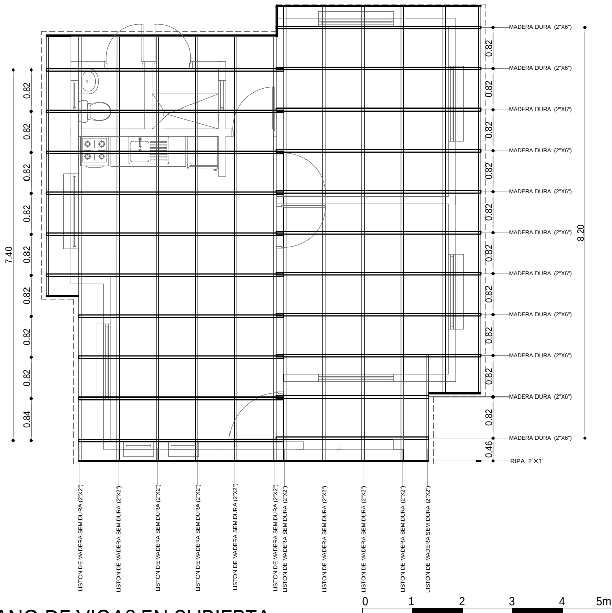
PLANO DE VIGAS EN CUBIERTA ESC. 1:75
