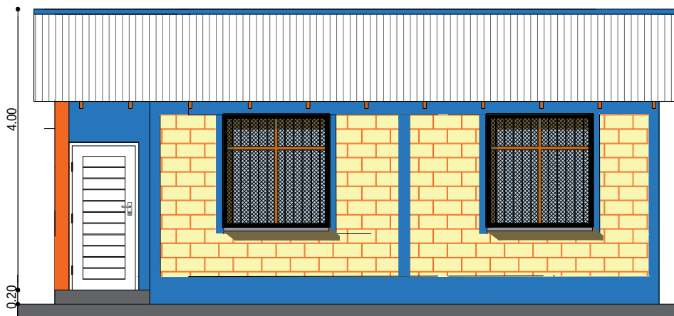
ELEVACION LATERAL ESC. 1:75
