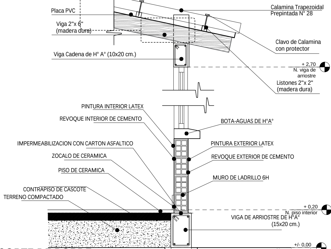
CORTE DE BORDE ESC. 1:20
