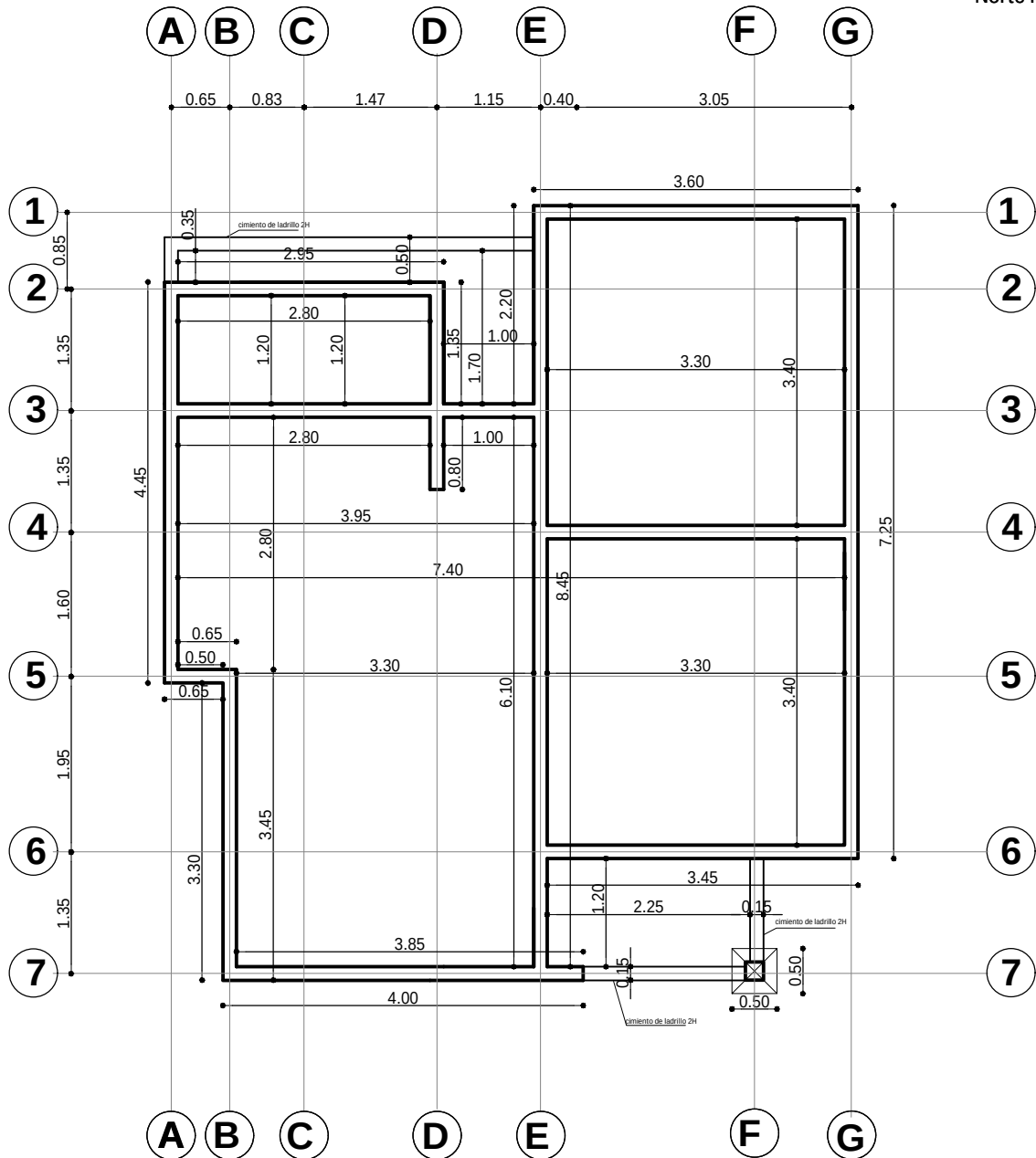
PLANO VIGA DE ARRIOSTRE ESC. 1:75
