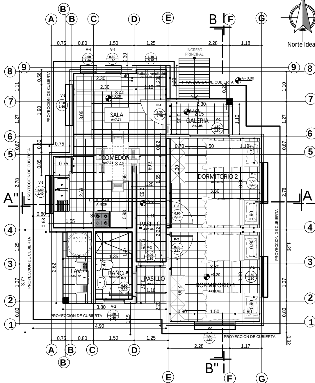
PLANTA ACOTADA ESC. 1:75
