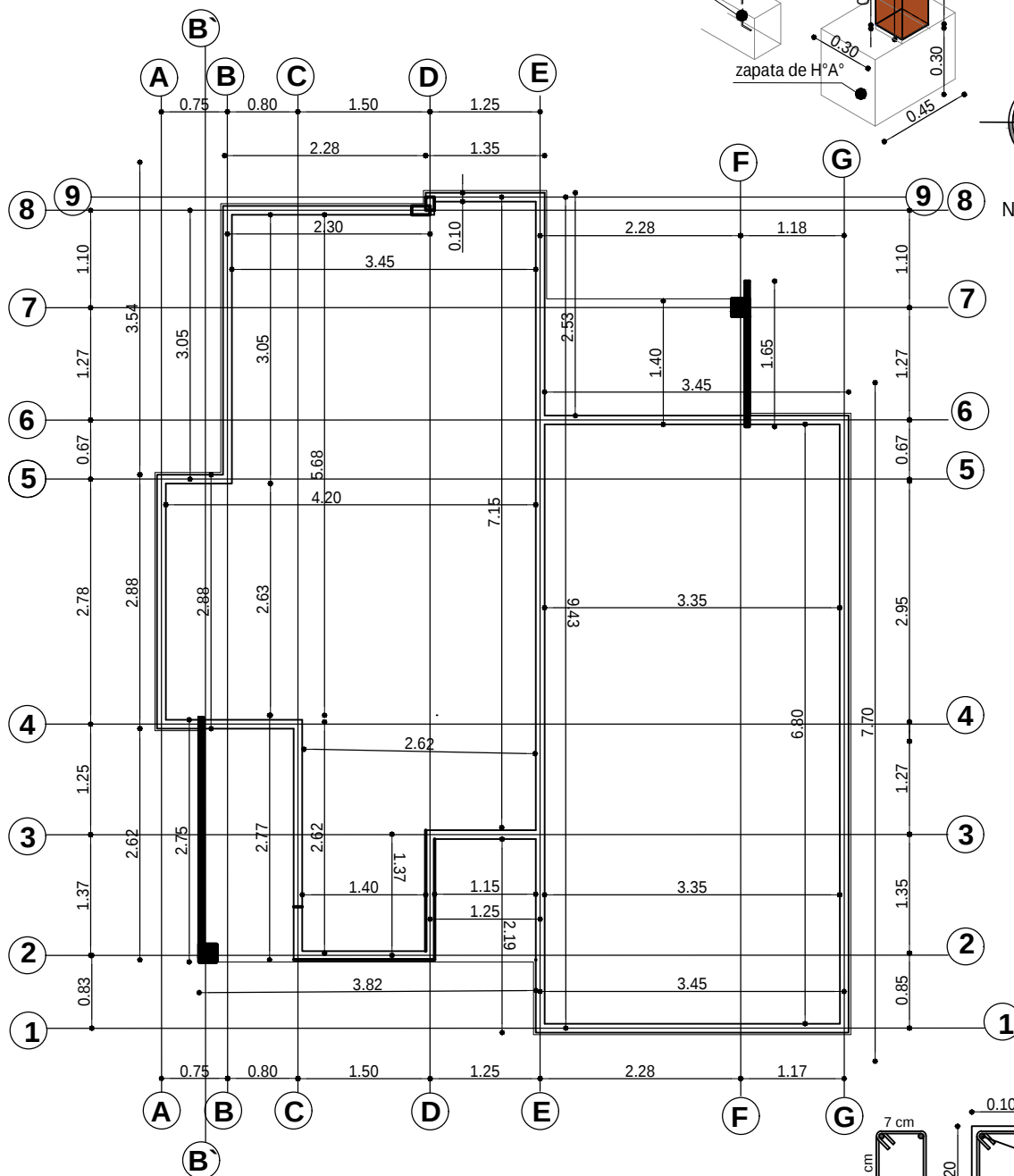
PLANO VIGA CADENA DE HºAº
