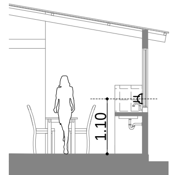
DETALLE ALTURA DE TOMACORRIENTES
