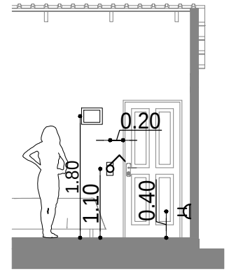
DETALLE ALTURA DE TOMACORRIENTES / INTERRUPTORES
