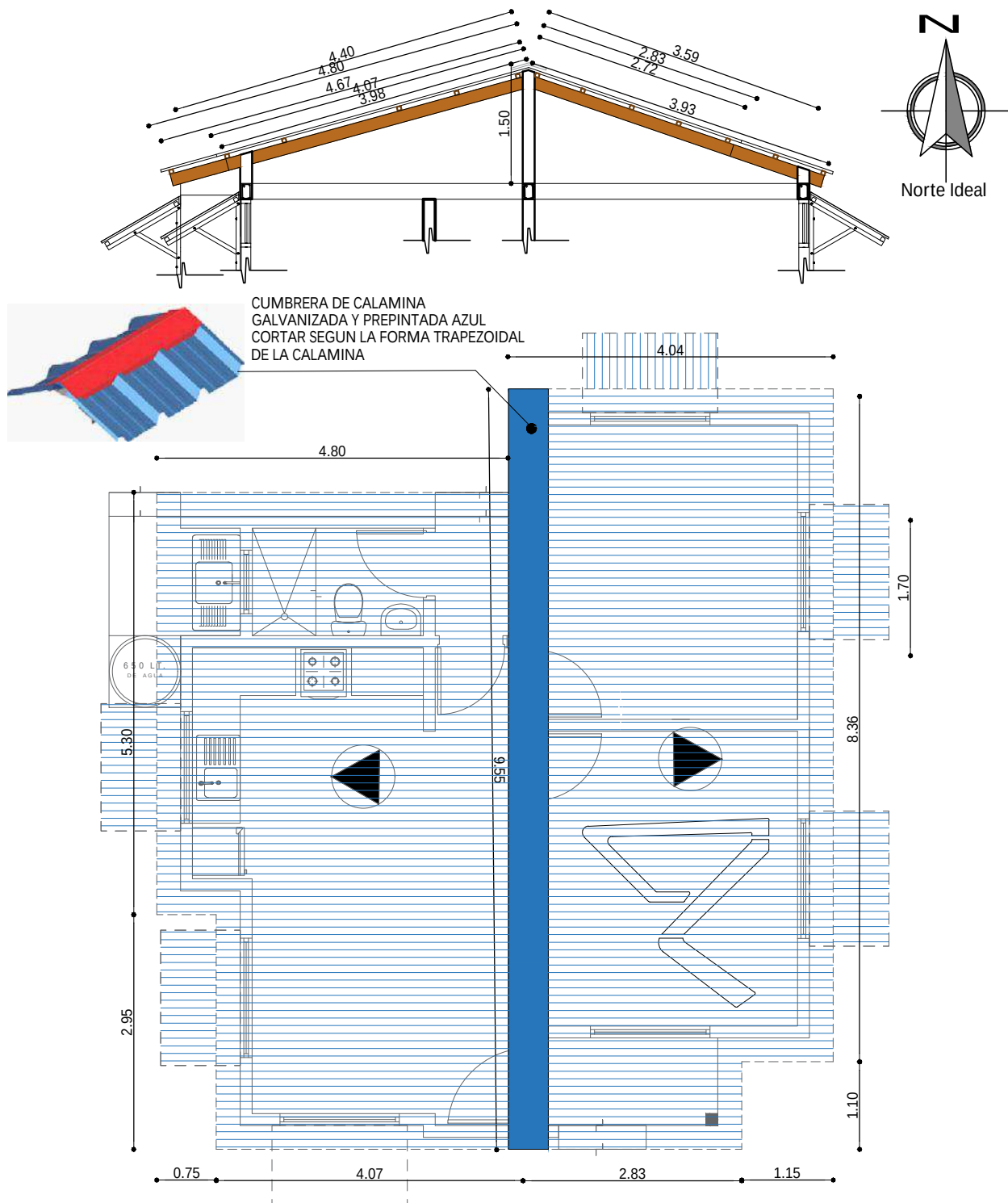
PLANO DE CUBIERTA ESC. 1:75
