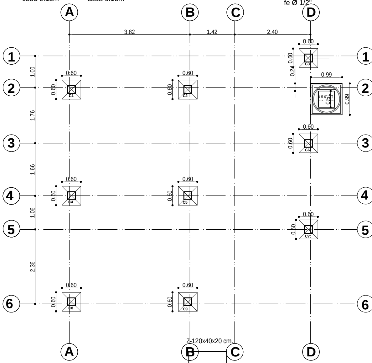
PLANO EXCAVACION-CIMIENTOS ESC. 1:75
