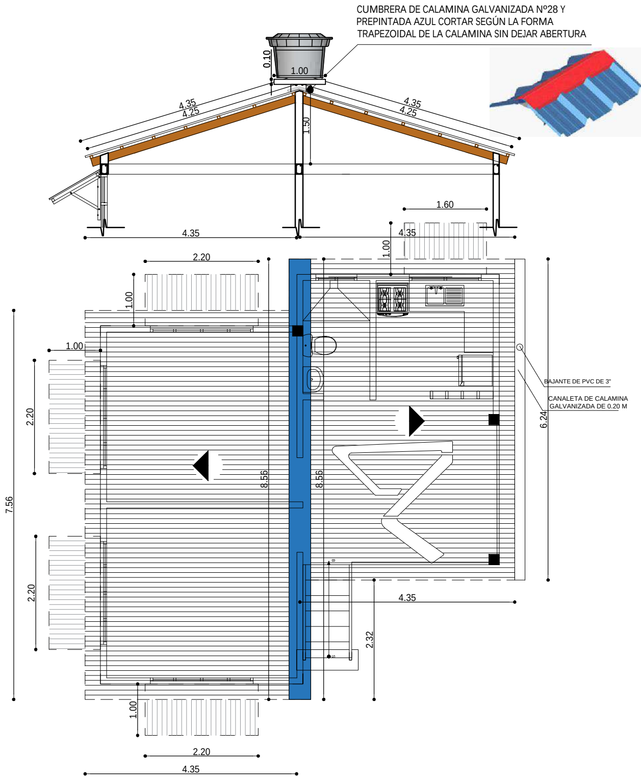
PLANO DE CUBIERTA ESC. 1:75
