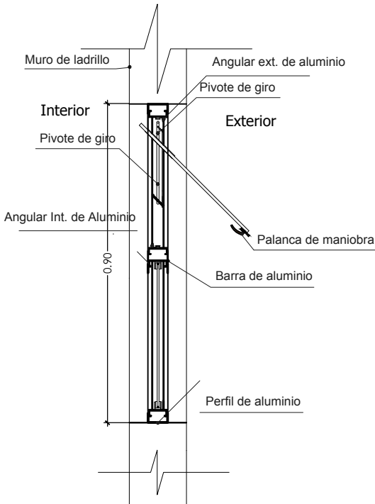
SECCION A-A
