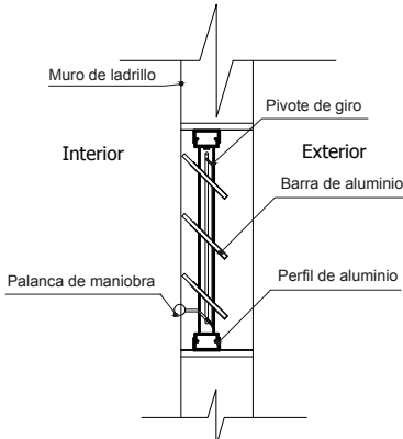
SECCION A-A
