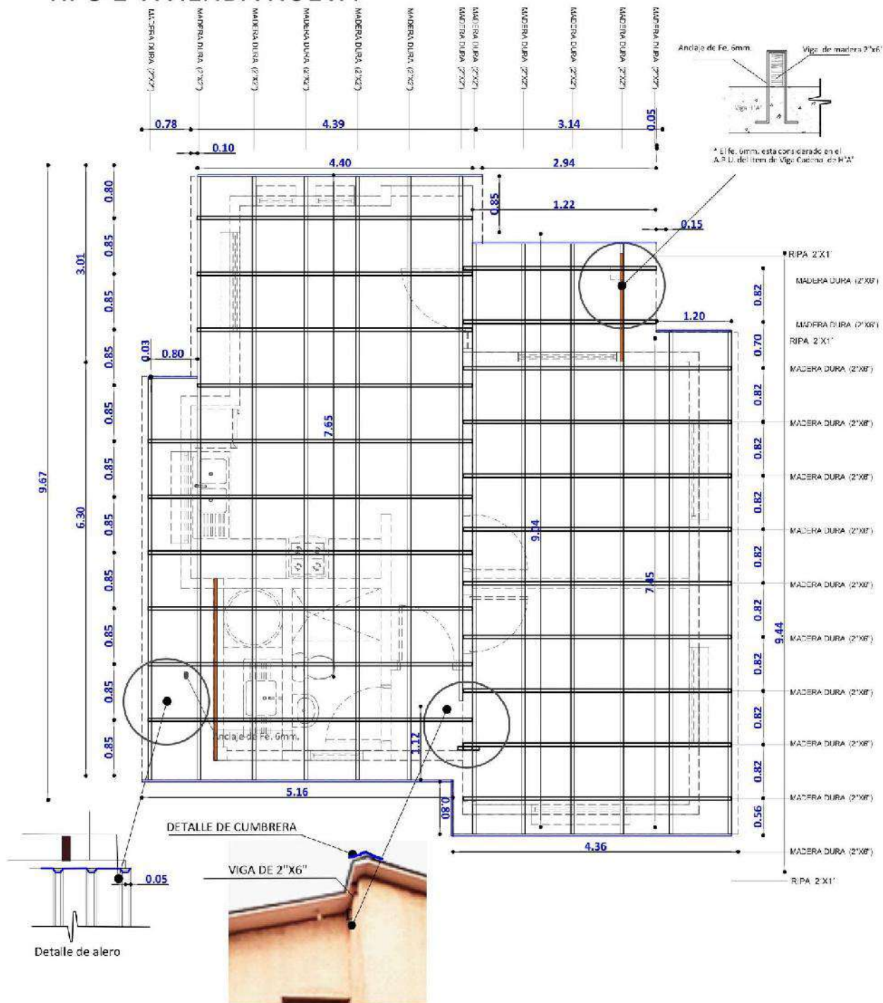
PLANO DE VIGAS EN CUBIERTA
