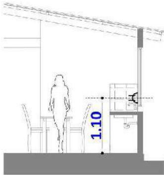
DETALLE ALTURA DE TOMACORRIENTE
