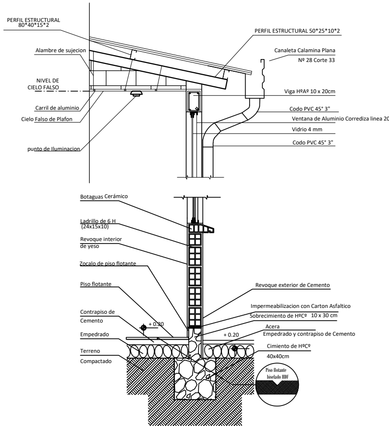
CORTE DE BORDE ESC. 1:30
