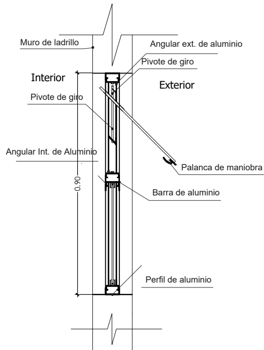
SECCION A-A
