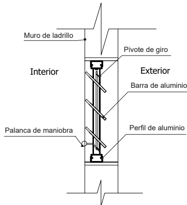
SECCION A-A
