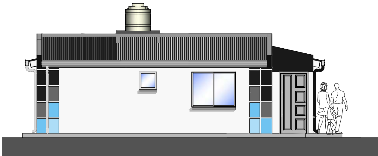
ELEVACION LATERAL
