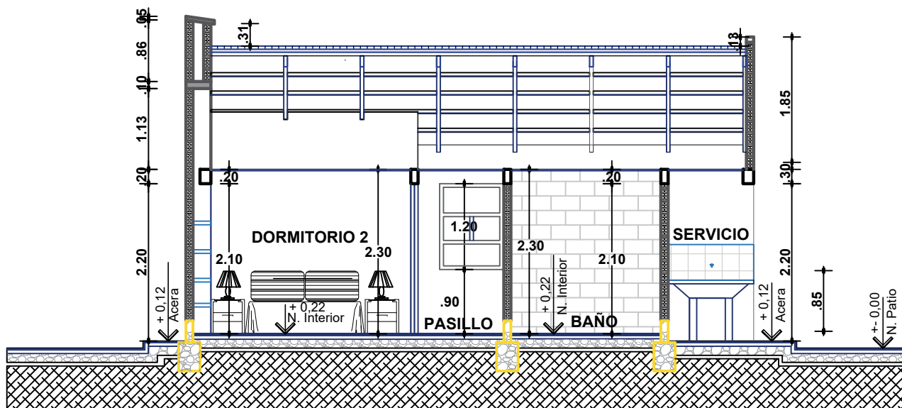
CORTE B-B'
