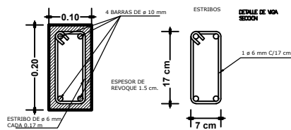
DETALLE DE VIGA 1
