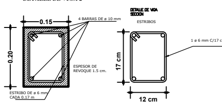
DETALLE DE VIGA 2
