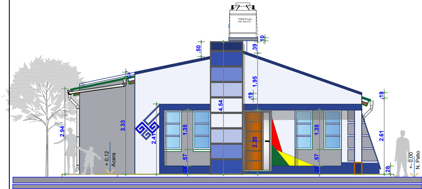
ELEVACION PRINCIPAL
