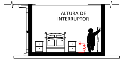
CORTE REFERENCIAL
