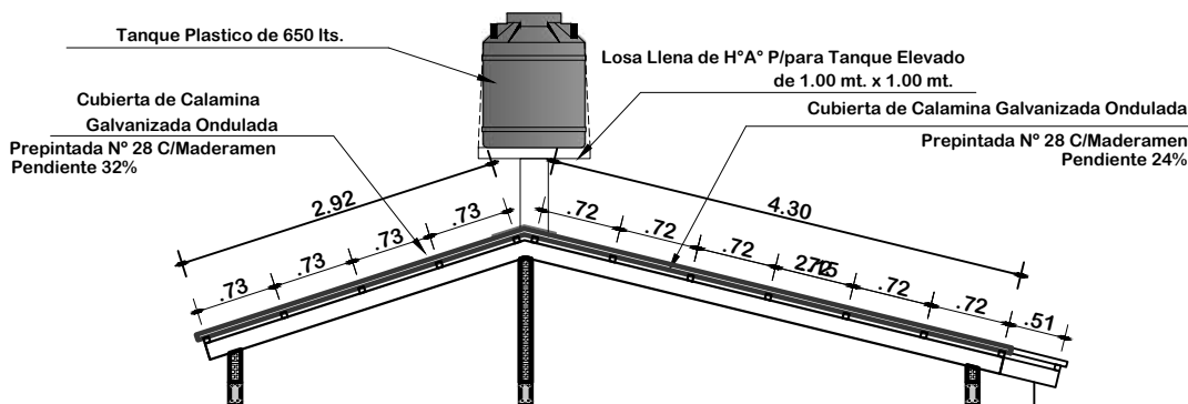
PLANO DE ESTRUCTURA MADERAMEN ESCALA: 1:75
