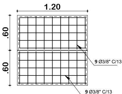
PLANTA
