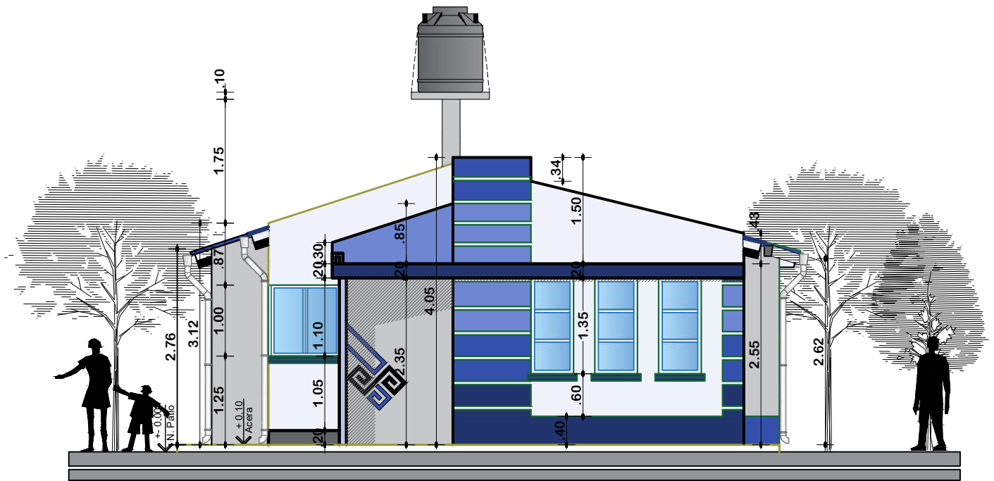
ELEVACION FRONTAL
