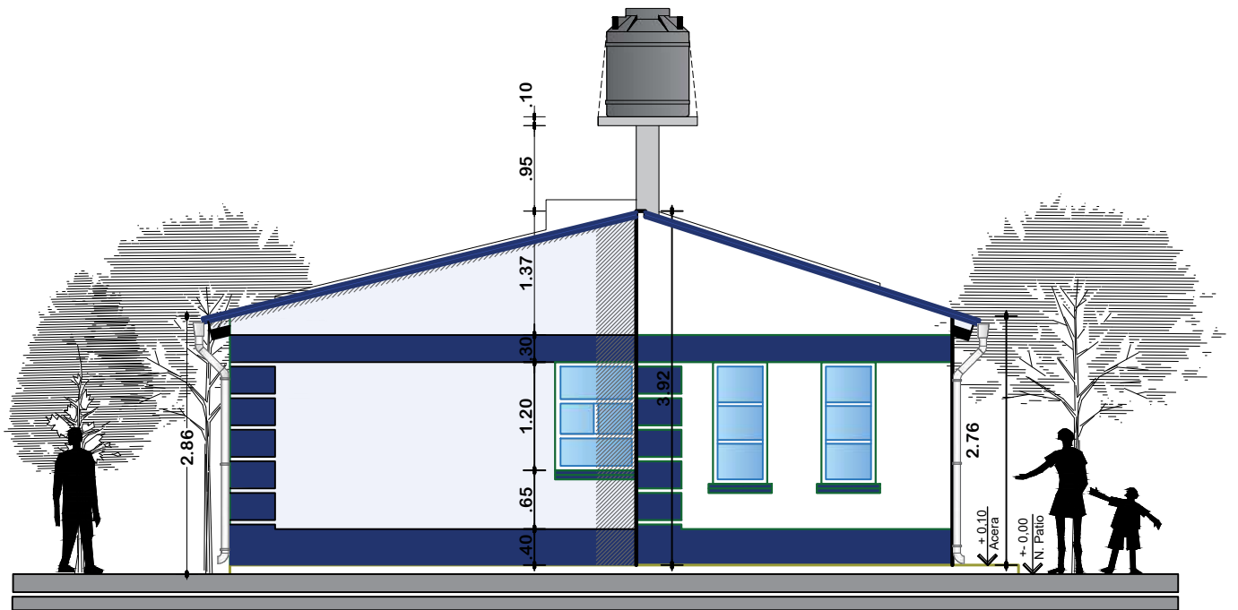
ELEVACION POSTERIOR
