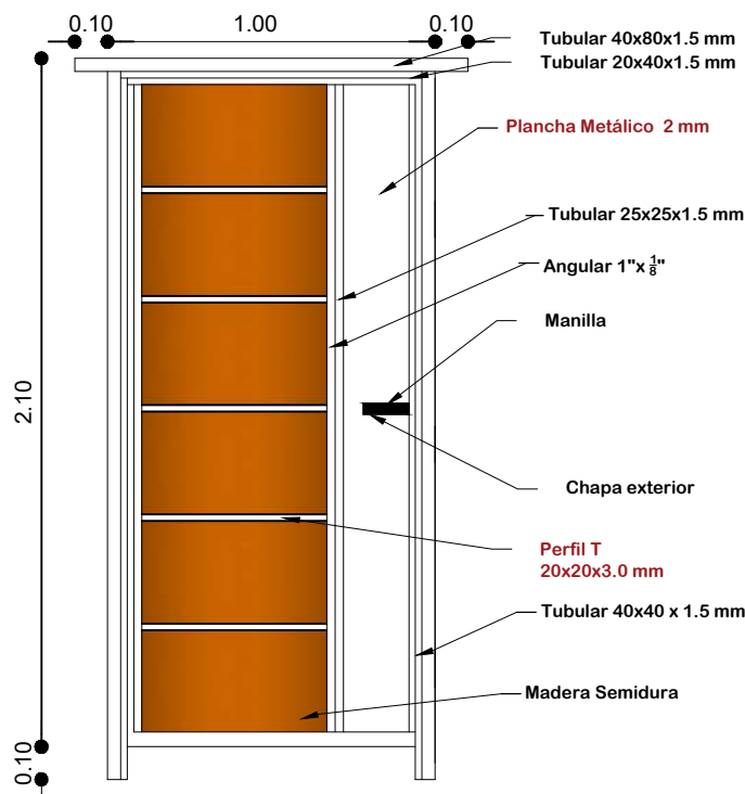
PUERTA 1.00 x 2,10
