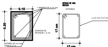
DETALLE DE VIGA 15x20
