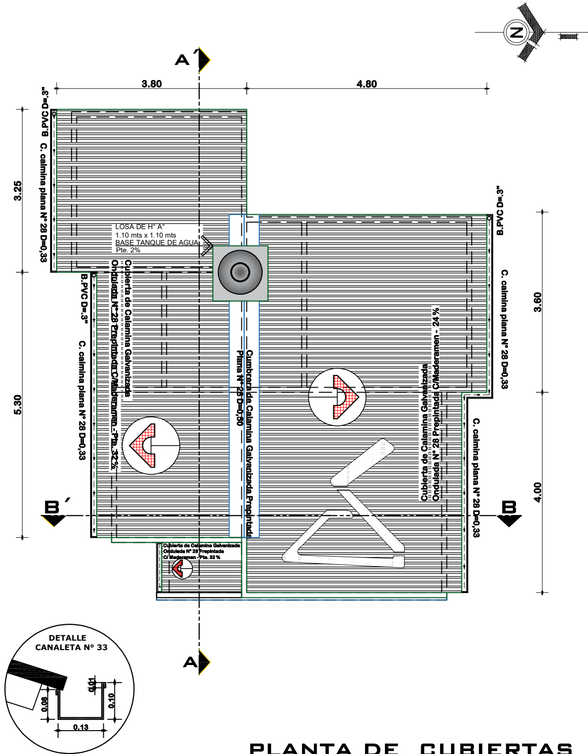
PLANTA DE CUBIERTAS ESCALA: 1:75
