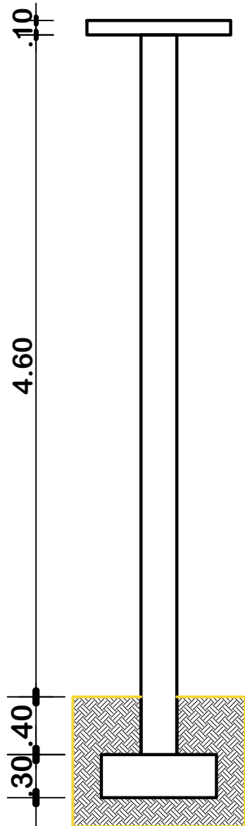
DETALLE COLUMNA DE HºAº Y ZAPATA DE HºAº ESCALA: 1:50
