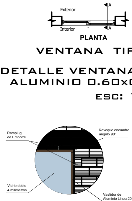
DETALLE VENTANA DE ALUMINIO LINEA 20 C/VIDRIO 4MM + ACCESORIOS
