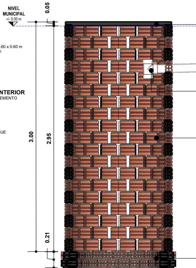
NIVEL MUNICIPAL +/- 0.00 m
