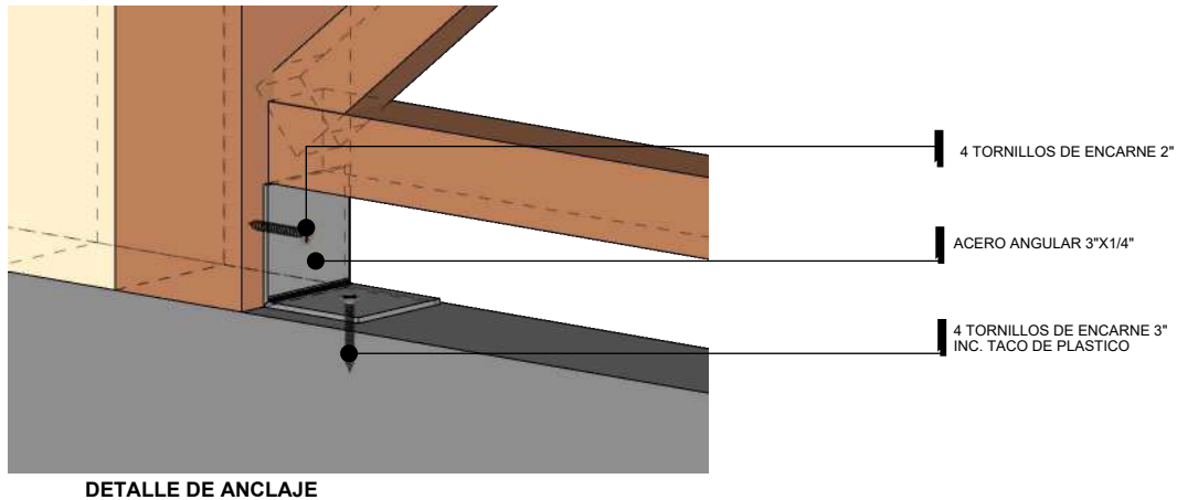
DETALLE DE ANCLAJE
