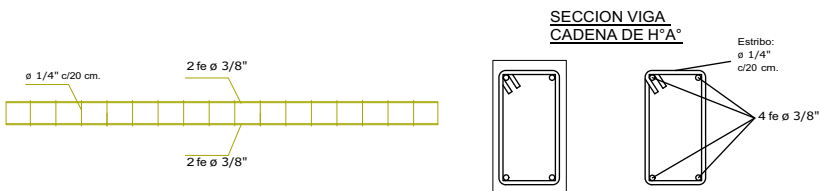
DETALLE VIGA DE 11º Aº
