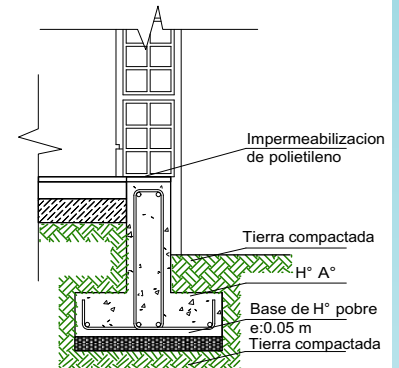
SECCION ESTRIBO
