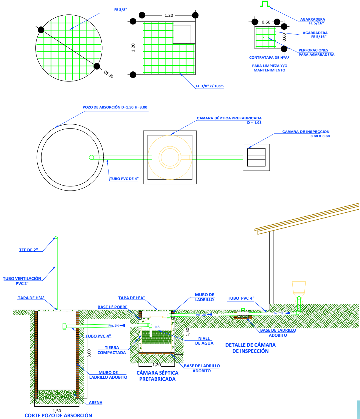
18 SISTEMA DE DESCARGA SANITARIO Scale: 1:75
