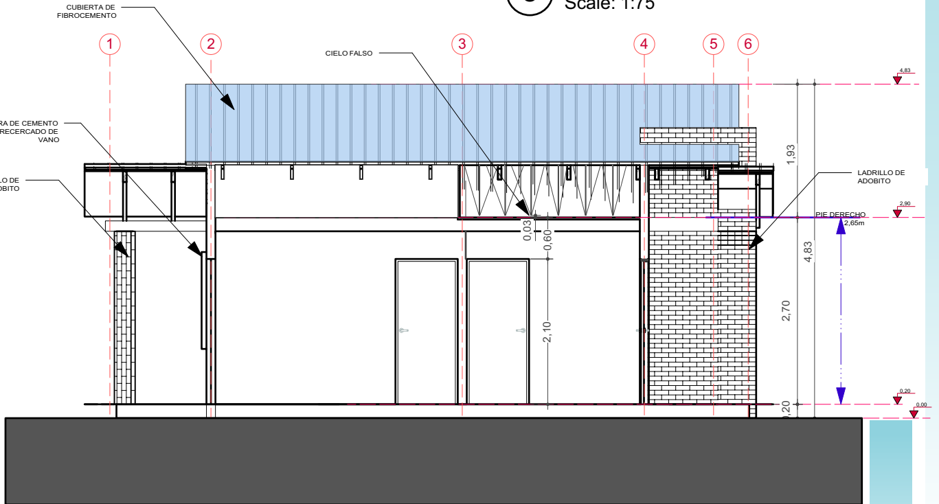
9 CORTE LONGITUDINAL B-B Scale: 1:75
