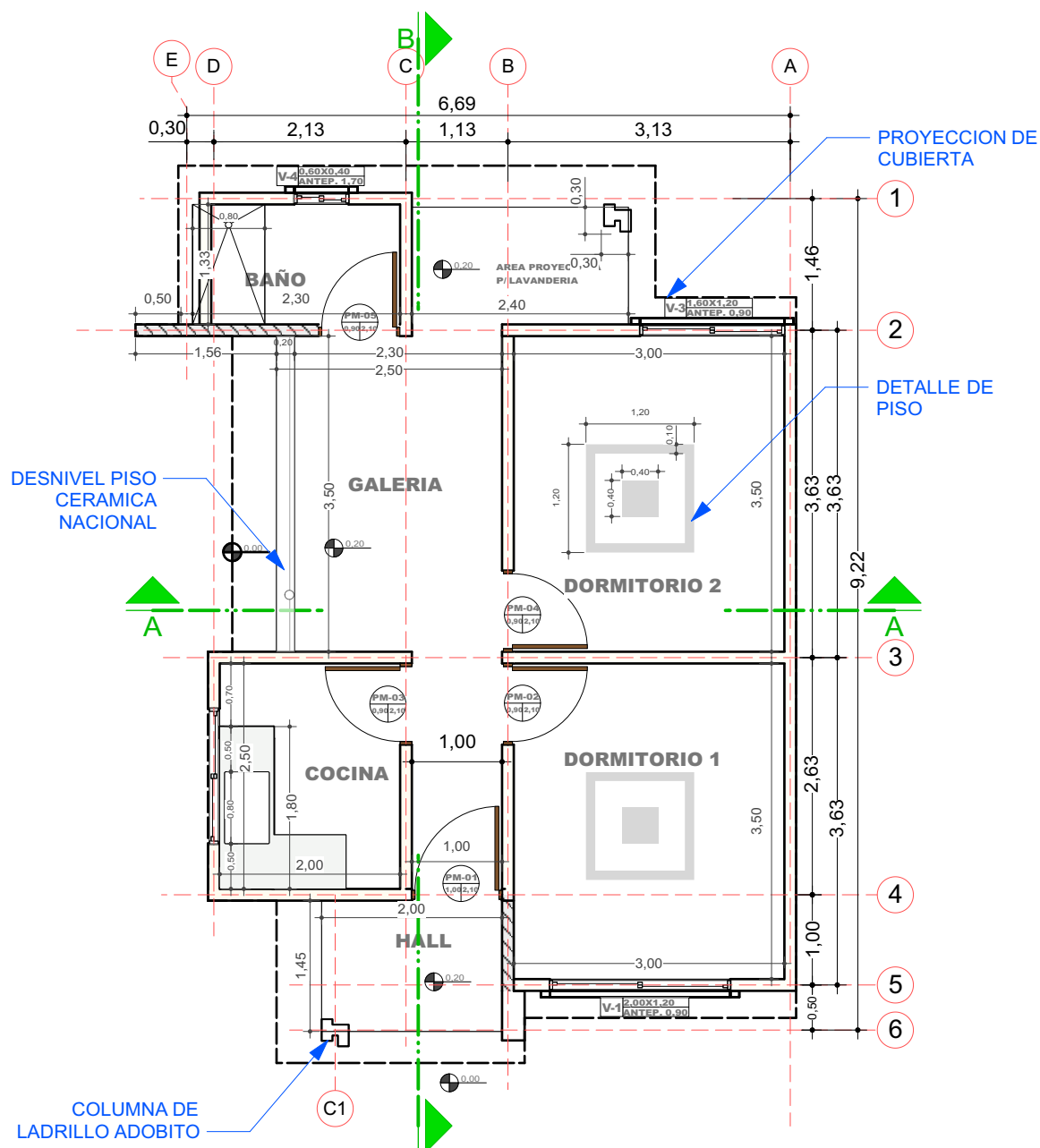
2 PLANO EN PLANTA - TECNICO
