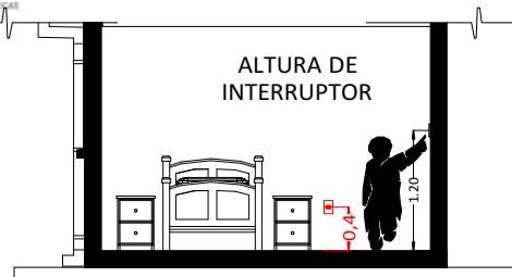
CORTE REFERENCIAL
