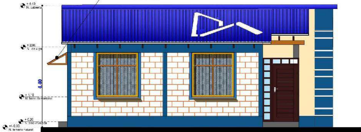
ELEVACION LATERAL DERECHA ESC. 1:75
