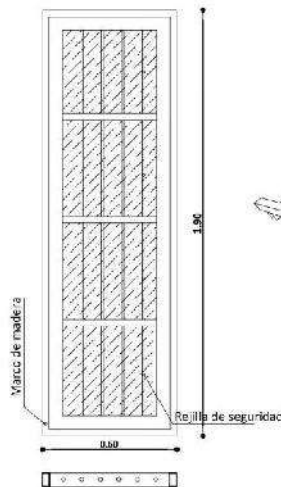
Ventana Tipo 4
