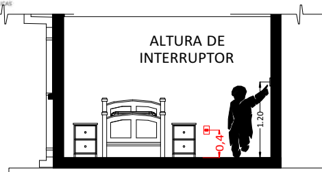
CORTE REFERENCIAL
