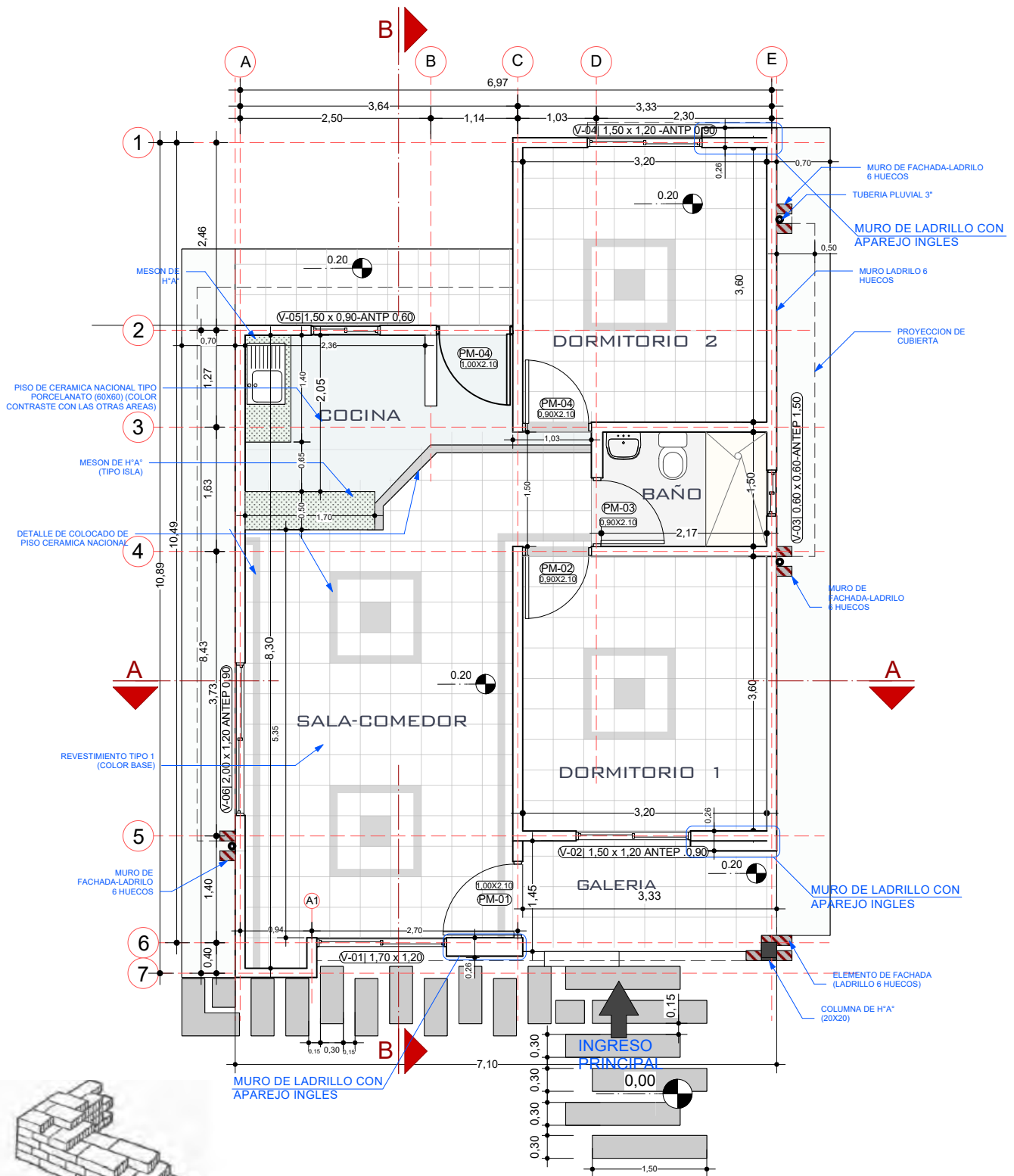
2 PLANO PLANTA TECNICA ACOTADA Escala: 1:75
