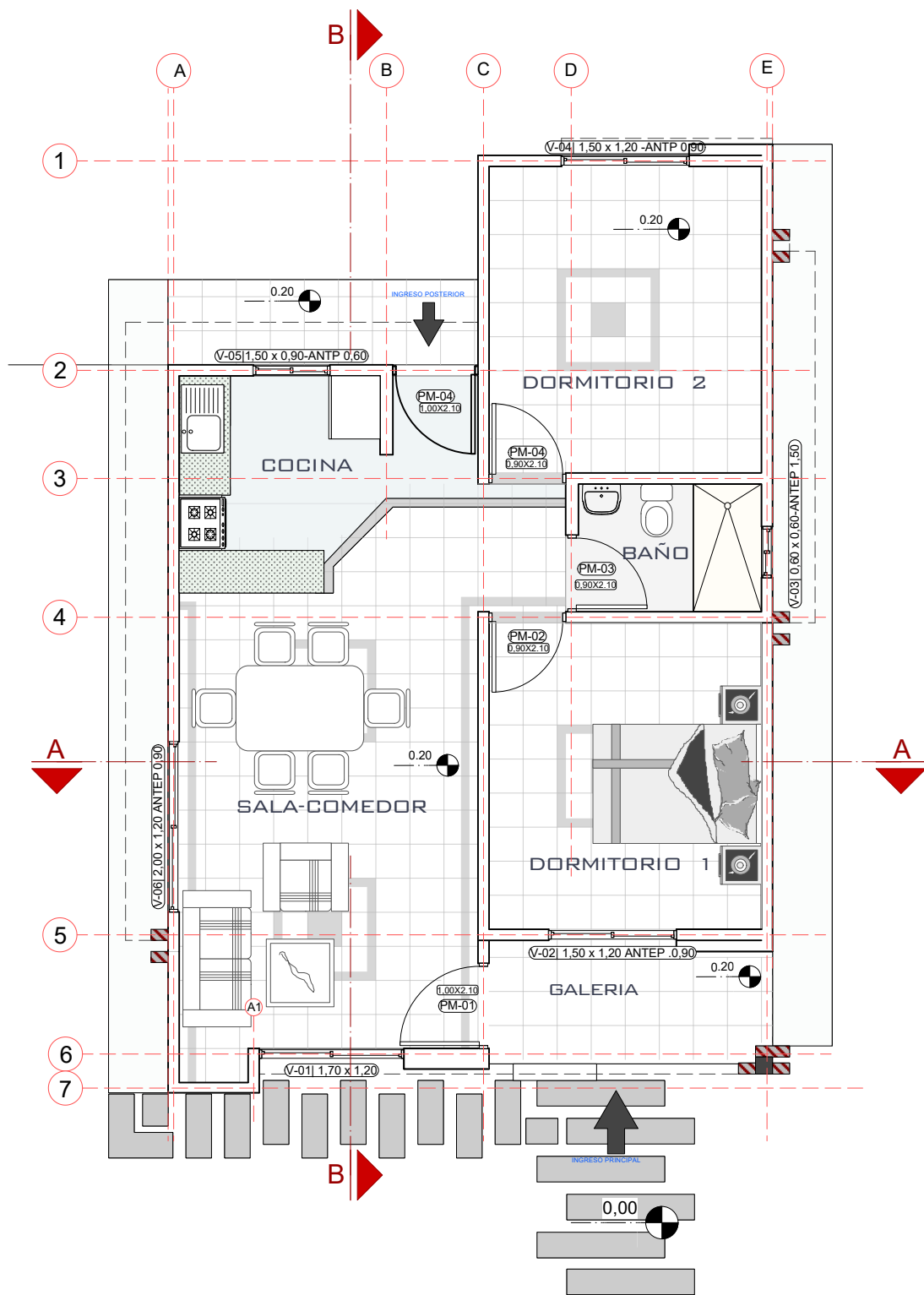
3 PLANO PLANTA AMOBLADA Escala: 1:75
