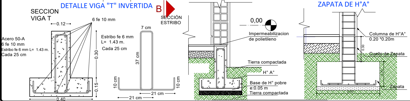
PLANO DE CIMIENTOS Escala: 1:75
