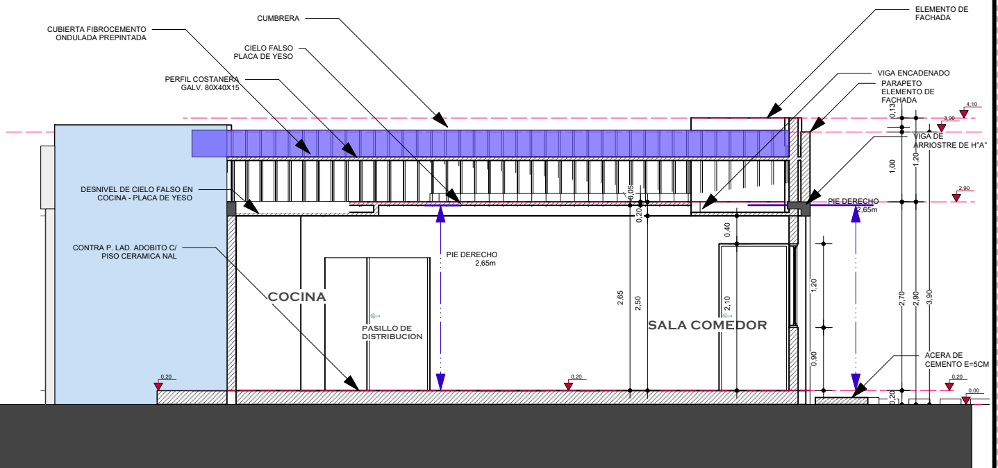
8 CORTE DE SECCION A-A' Escala: 1:75
