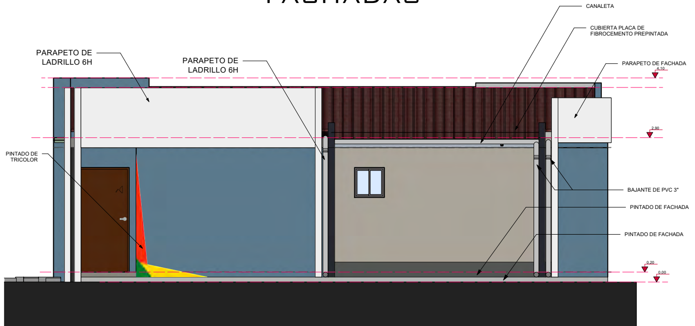
12 FACHADA LATERAL DERECHA Escala: 1:75
