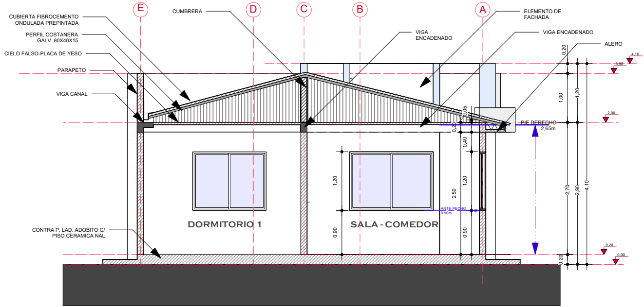
8 CORTE DE SECCION A-A' Escala: 1:75
