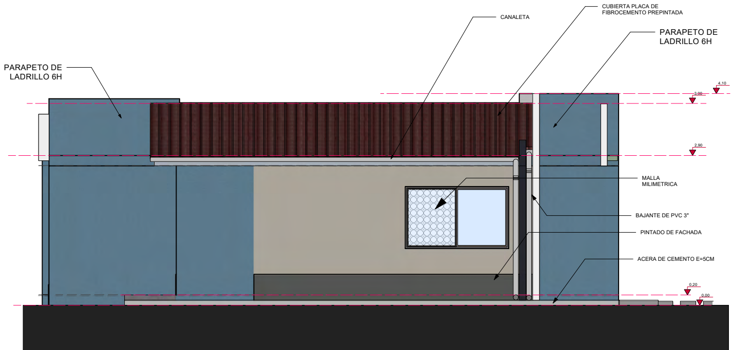
12 FACHADA LATERAL DERECHA Escala: 1:75
