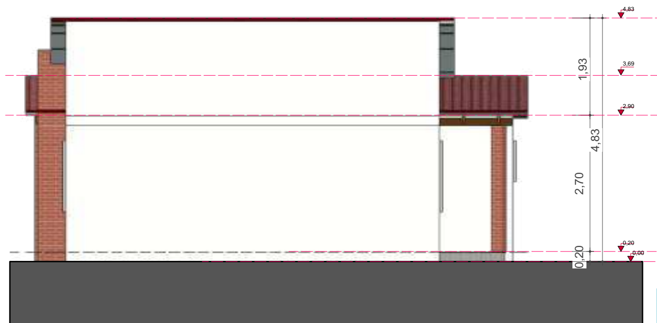
FACHADA LATERAL DERECHA Scale: 1:75
