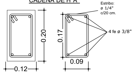
DETALLE VIGA DE H°A°
