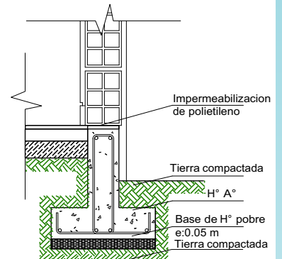
SECCI3N ESTRIBO
