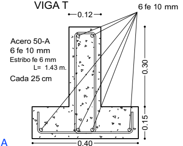
SECCION VIGA T
