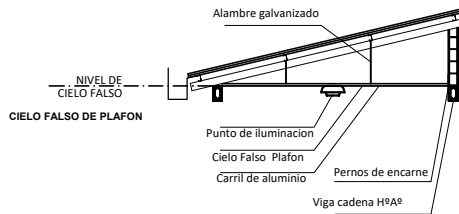
CORTE DE BORDE ESC. 1:30
