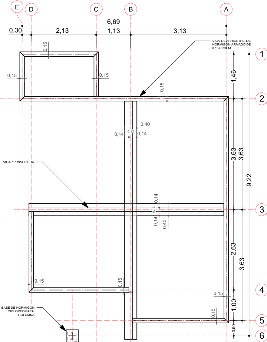
1 PLANO DE CIMENTACION Scale: 1:75
