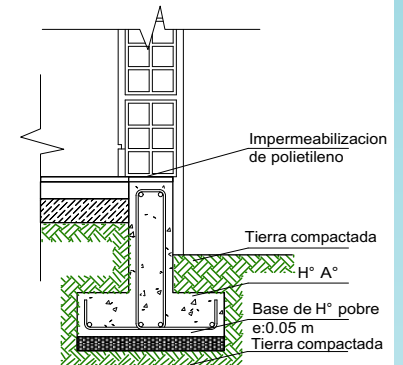
SECCIÓN ESTRIBO
