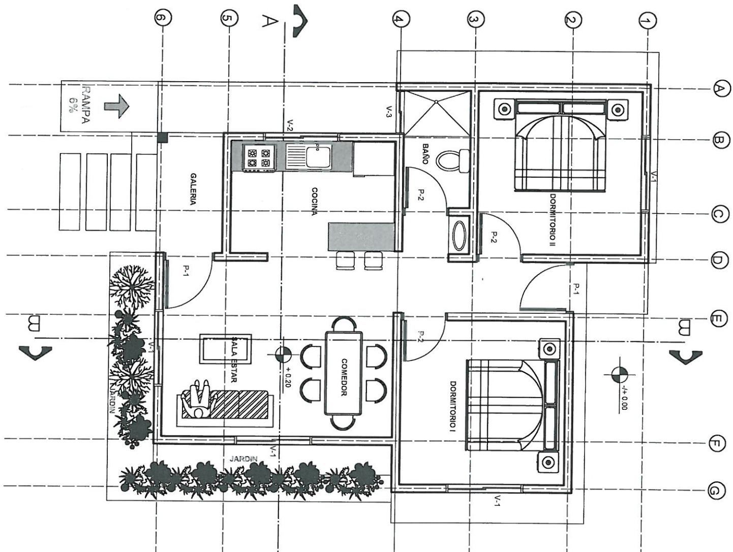
PLANTA AMOBLADA GENERAL ESC 1:75
