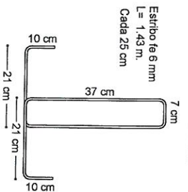
SECCIÓN ESTRIBO
