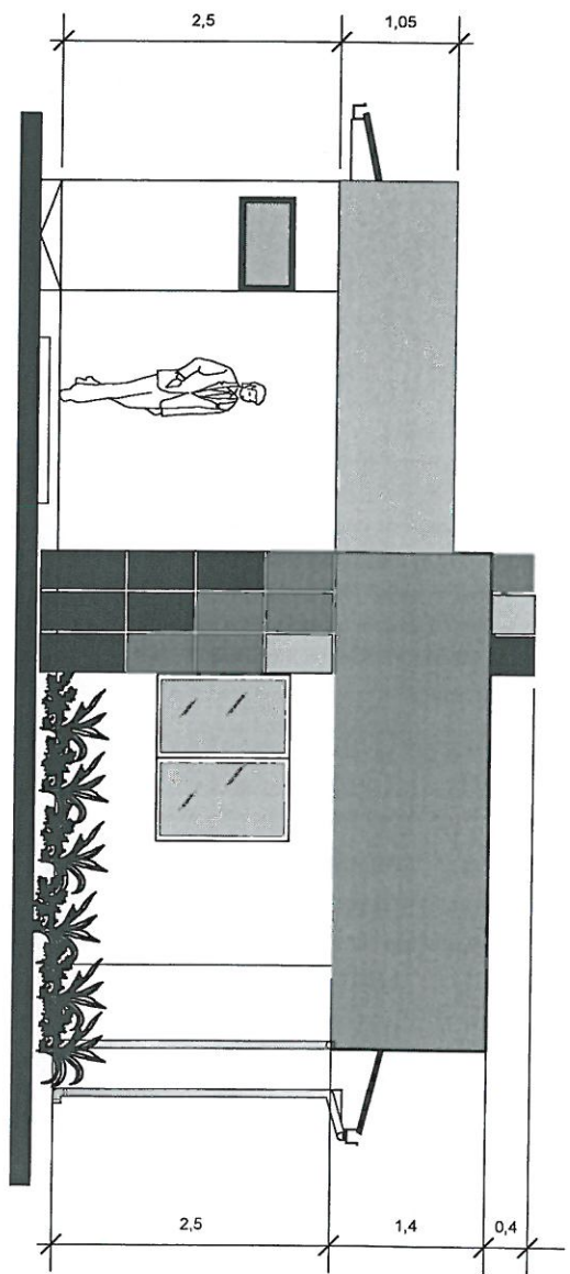
FACHADA FRONTAL ESC.: 1:75
