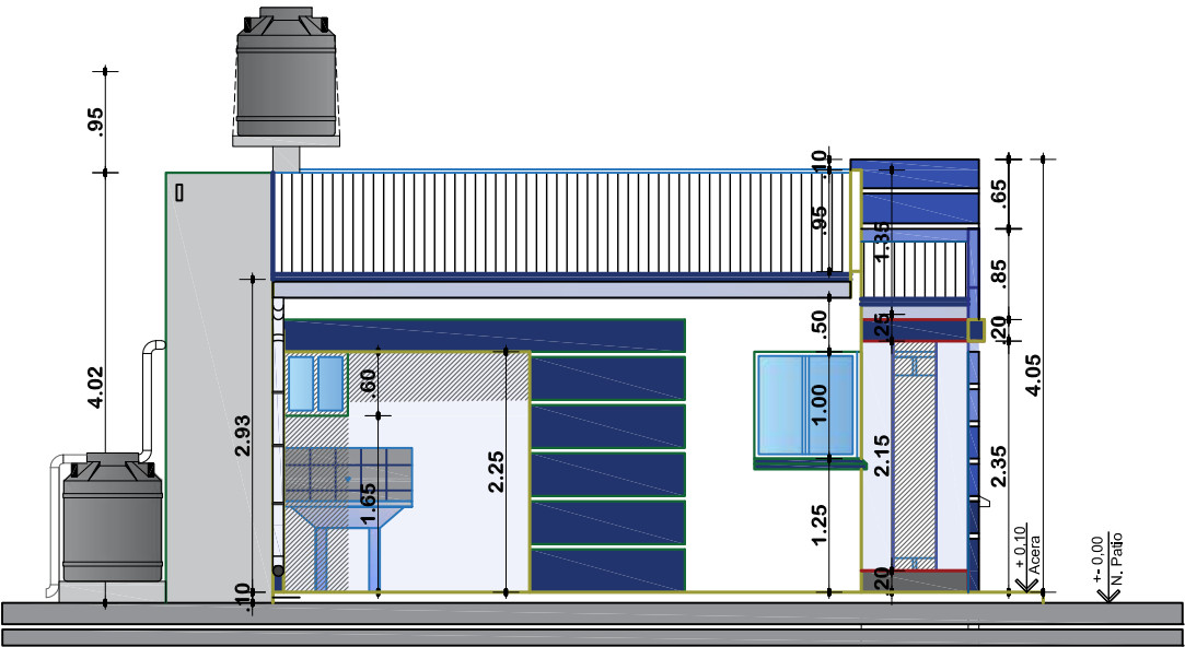
ELEVACION LATERAL DERECHO ESCALA: 1:75
