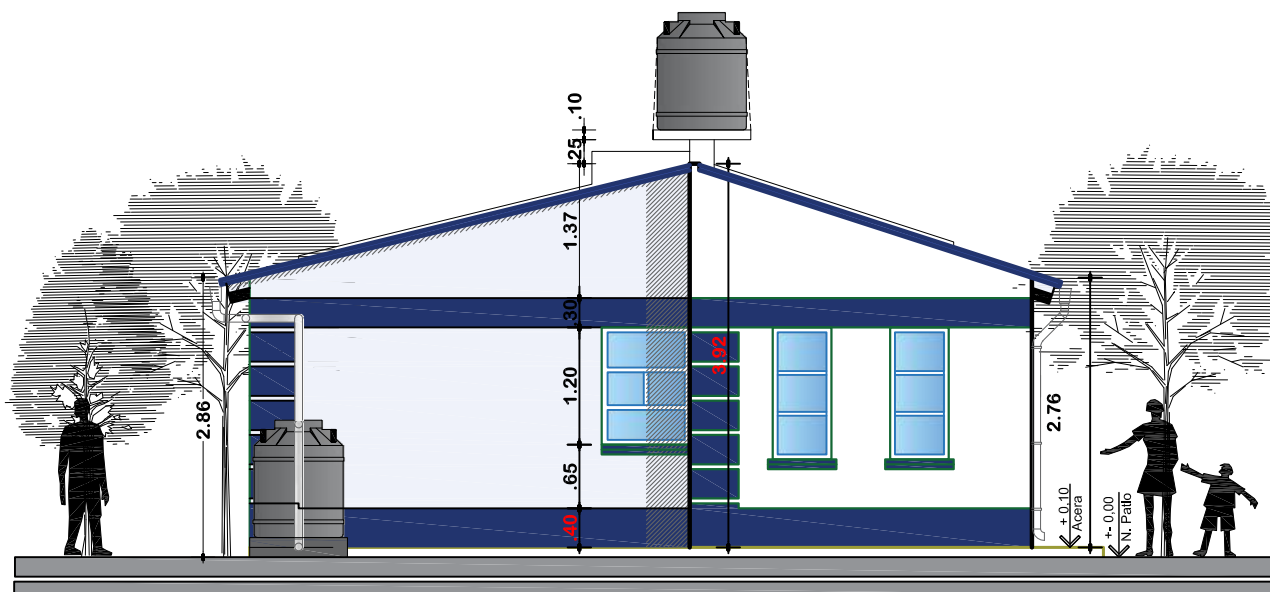
ELEVACION POSTERIOR ESCALA: 1:75
