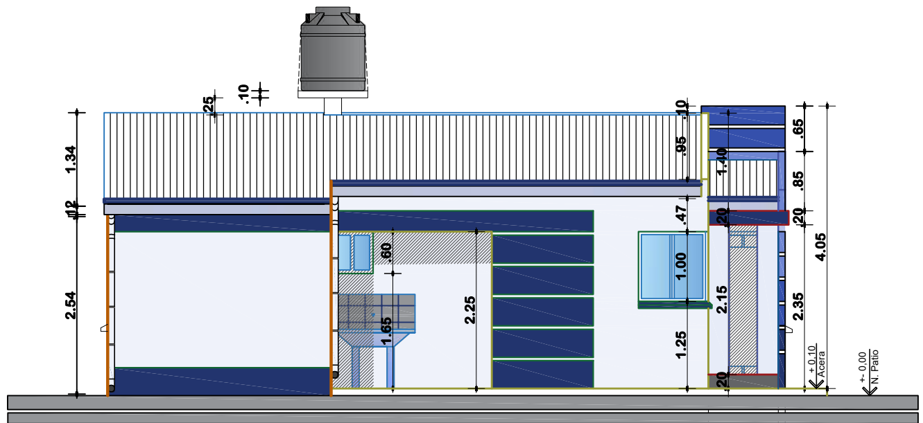
ELEVACION LATERAL DERECHO ESCALA: 1:75
