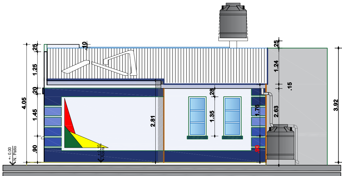
ELEVACION LATERAL IZQUIERDO ESCALA: 1:75
