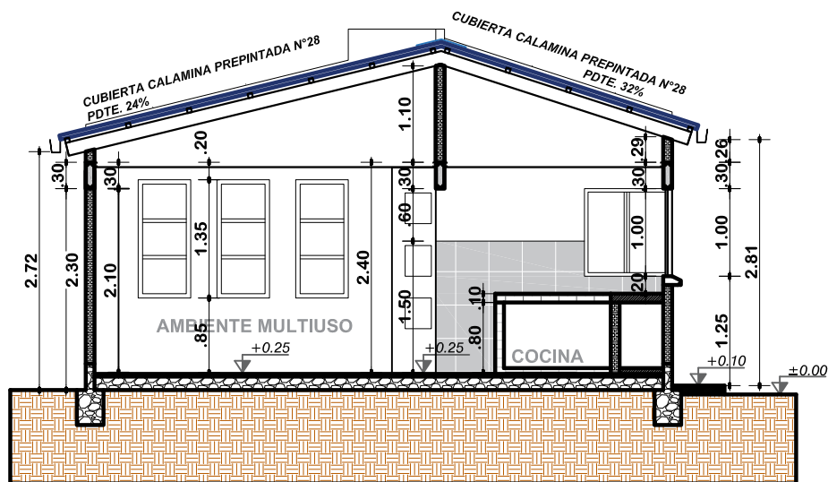
CORTE B-B' ESCALA: 1:75
