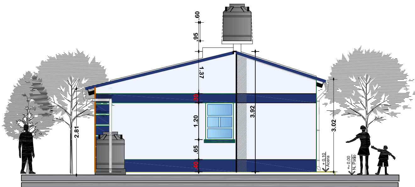
ELEVACION POSTERIOR ESCALA: 1:75
