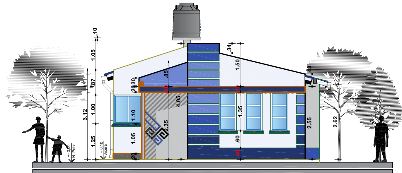
ELEVACION FRONTAL ESCALA: 1:75
