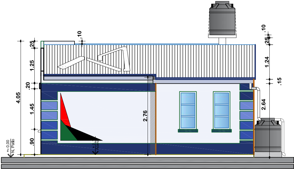
ELEVACION LATERAL IZQUIERDO ESCALA: 1:75
