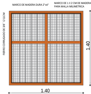
Ventana Tipo 1
