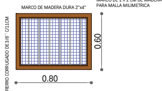
Ventana Tipo 3
