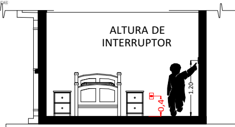
CORTE REFERENCIAL
