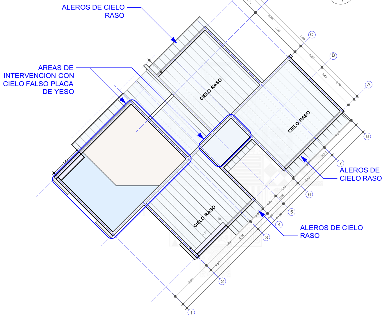
6 PLANO DE UBICACION / CIELO FALSO Y RASO Scale: 1:100
