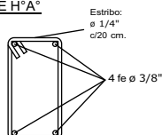
4 PLANO DE VIGA DE ENCADENADO Scale: 1:100
