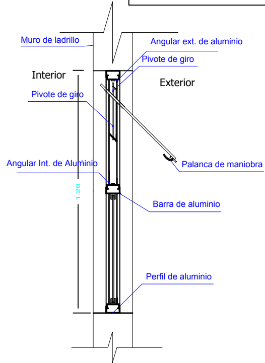
SECCION A-A
