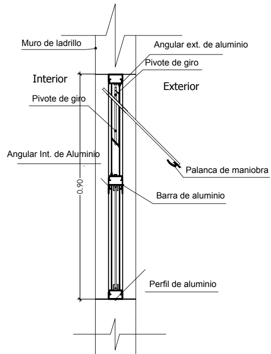
SECCION A-A
