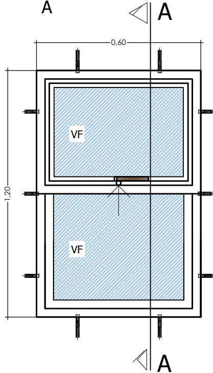
ELEVACION
