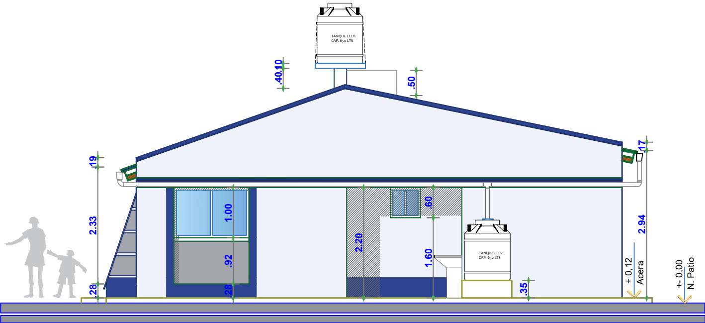
ELEVACION POSTERIOR ESC. 1:75
