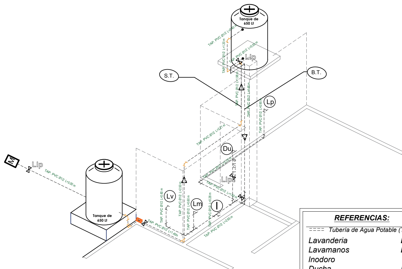
ISOMETRIA ESCALA: 1:75
