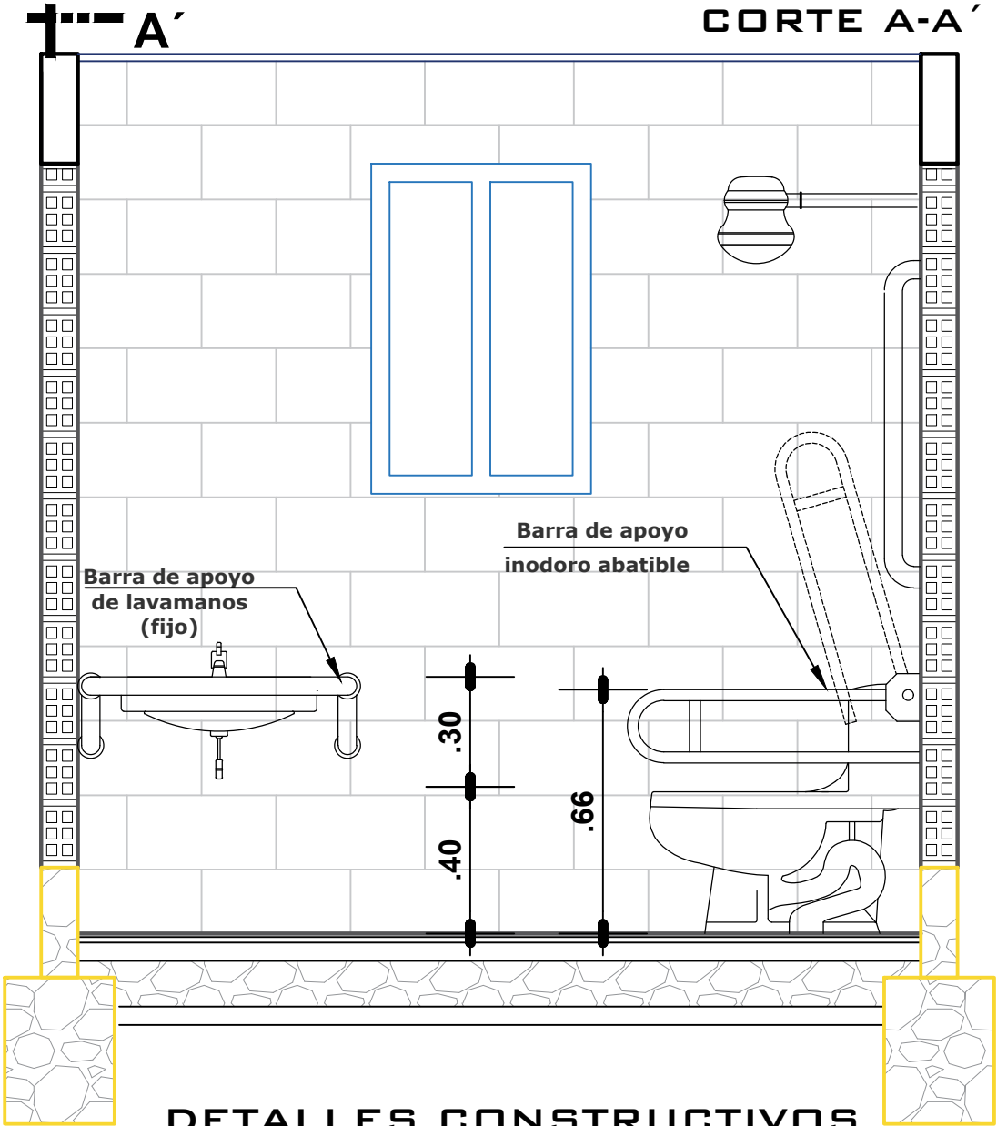
DETALLES CONSTRUCTIVOS BAÑO ESCALA: 1:25
