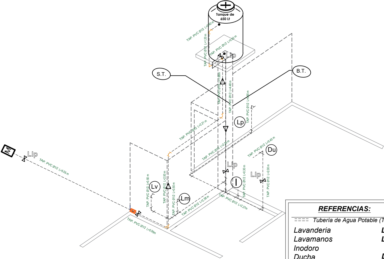
ISOMETRIA ESCALA: 1:75
