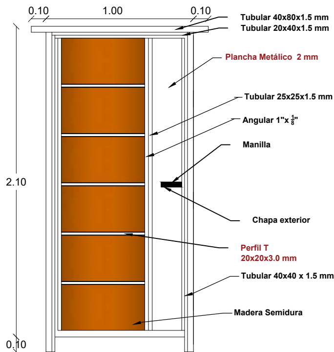
PUERTA 1.00 x 2,10
