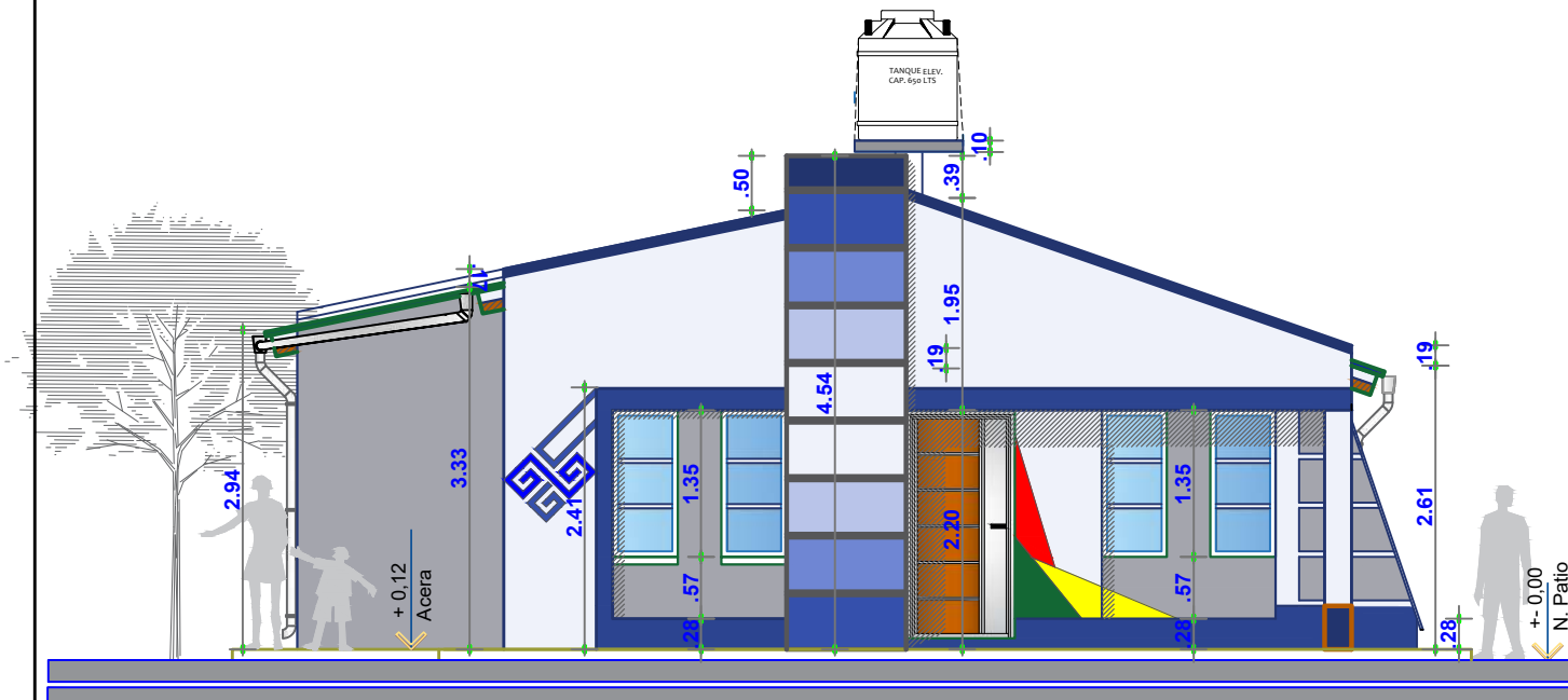
ELEVACION PRINCIPAL
