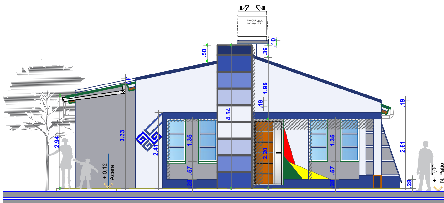
ELEVACION PRINCIPAL
