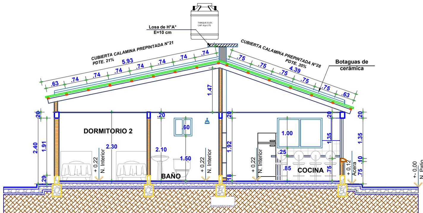
CORTE A-A'
