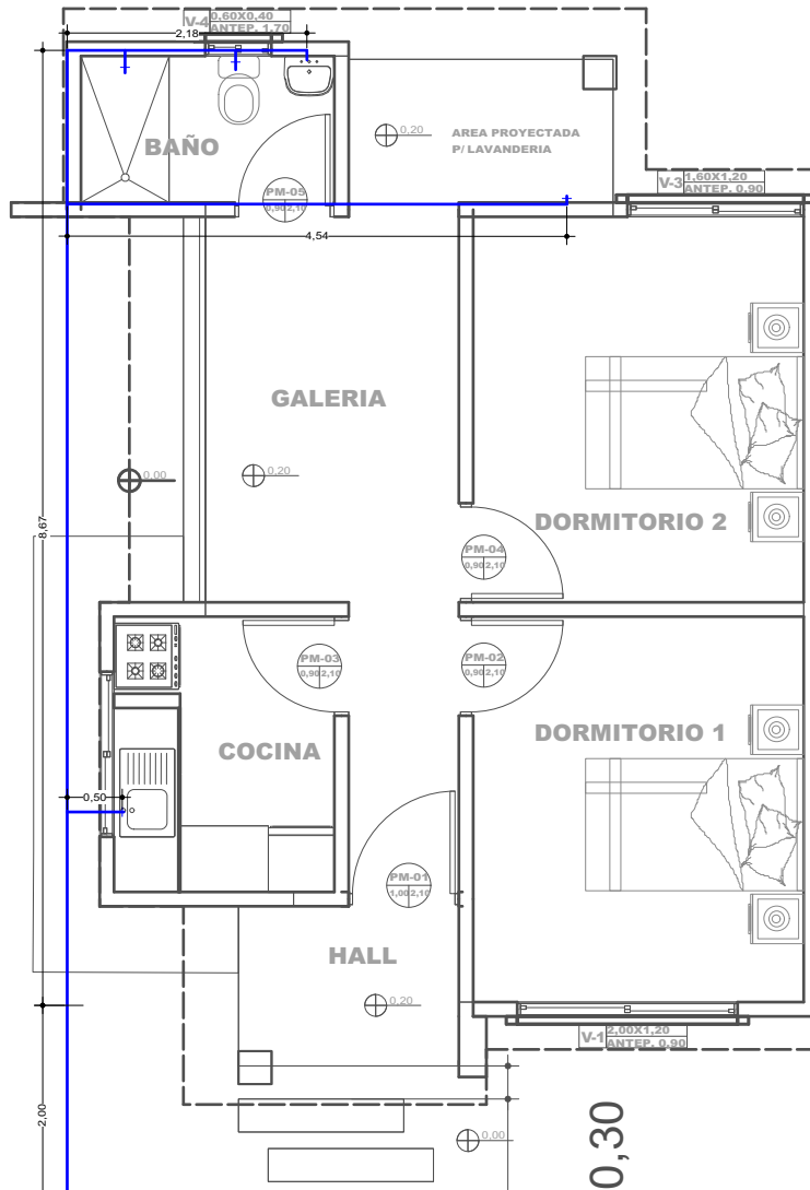
PLANO DE INSTALACIONES HIDRAULICAS Scale: 1:75
