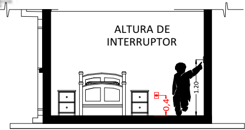
CORTE REFERENCIAL
