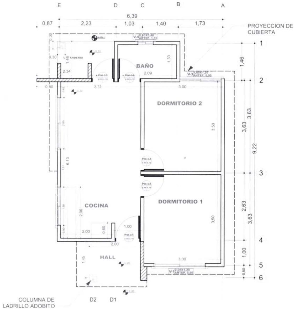
2 PLANO EN PLANTA - TECNICO Scale: 1:75
