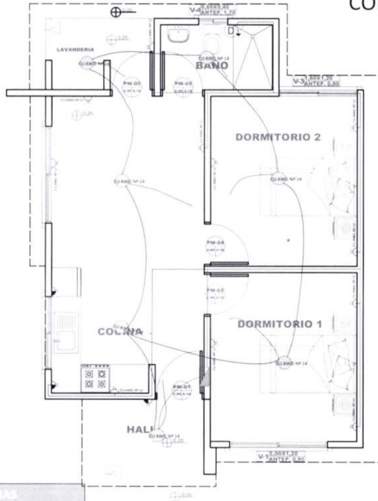
14 PLANO DE INSTALACIONES ELECTRICAS Scale: 1:75
