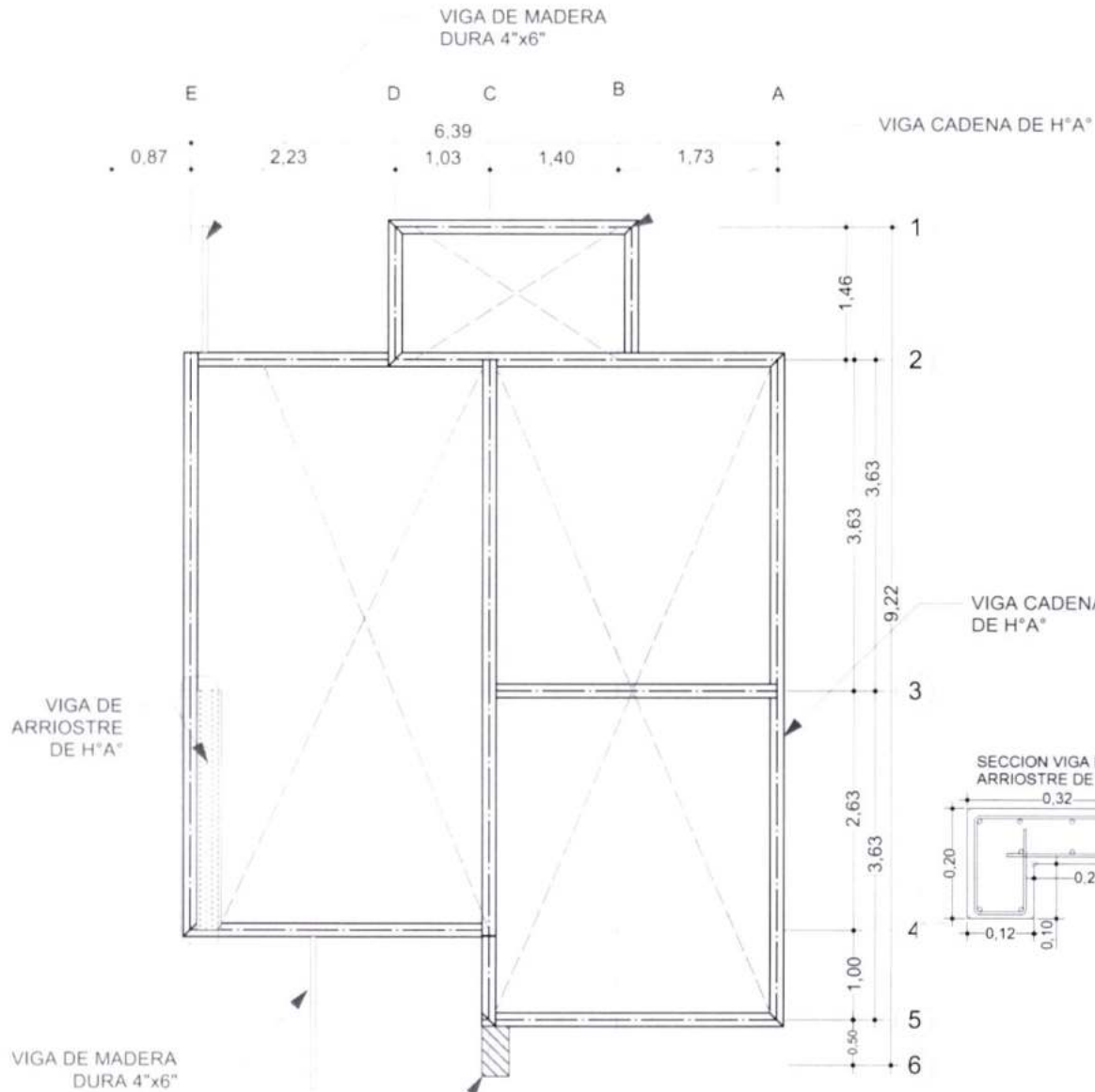
4 PLANO DE VIGA ENCADENADO Scale: 1:75
