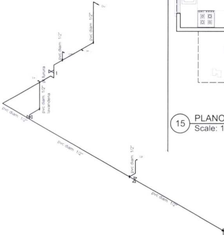
40 PLANO ESQUEMATICO ISOMETRICO - DE INSTALACION HIDRAULICA Scale: 1:100
