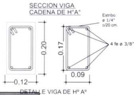
4 PLANO DE VIGA ENCADENADO Scale: 1:75
