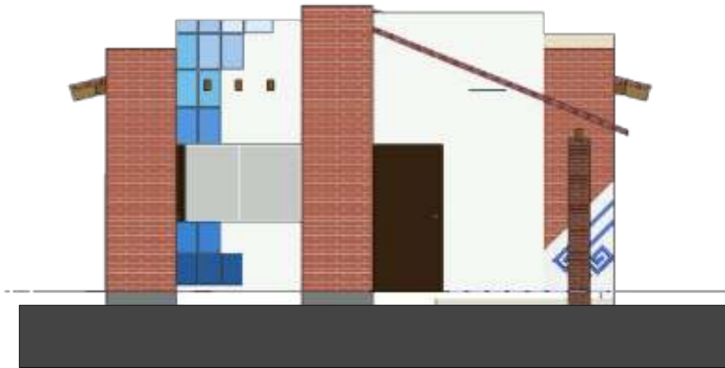
11 FACHADA FRONTAL Scale: 1:75
