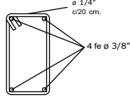
SECCION VIGA CADENA DE H'A°
