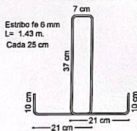
SECCION VIGA T
