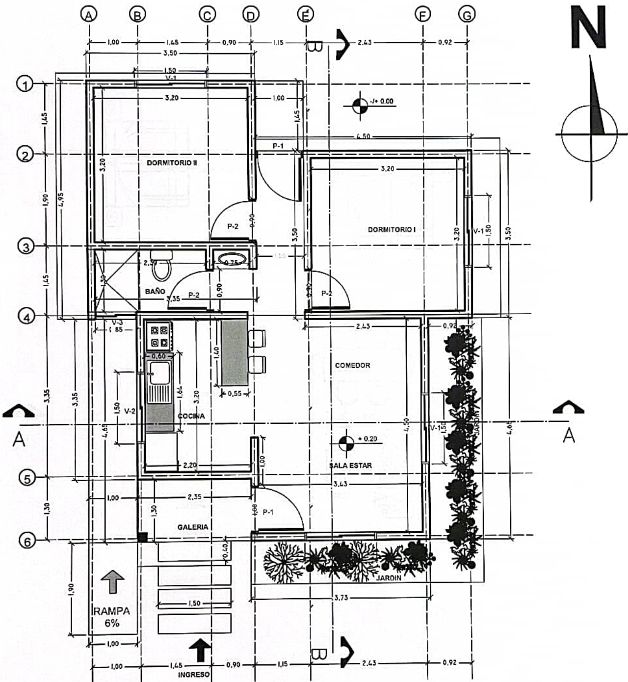
PLANTA ACOTADA GENERAL ESC.: 1:75
