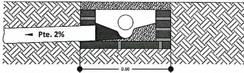
DETALLE CÁMARA DE INSPECCIÓN (0,60 x 0,60)
