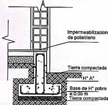
SECCIÓN ESTRIBO
