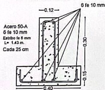
SECCION VIGA T
