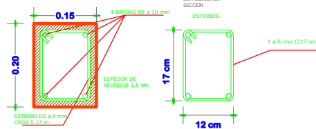
DETALLE DE VIGA 15x20
