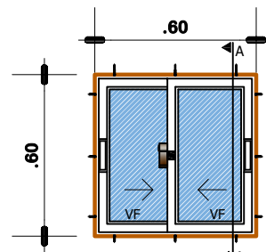
ELEVACION
