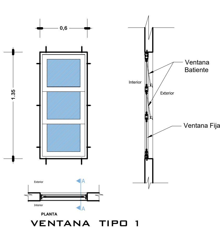
DETALLE VENTANA DE ALUMINIO 0.60x1.35
