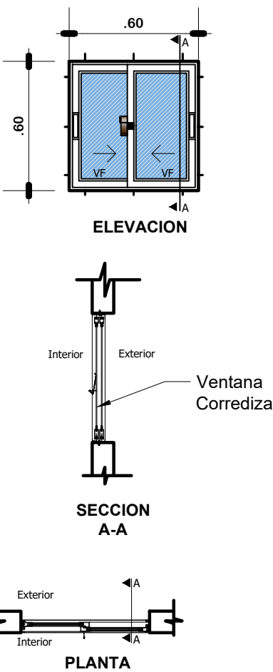
DETALLE VENTANA DE ALUMINIO 0.60x0.60
