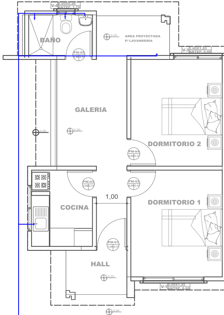
PLANO DE INSTALACIONES HIDRAULICAS Scale: 1:75
