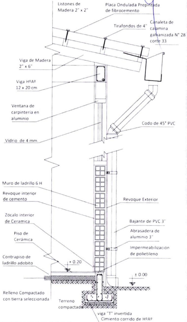
CORTE DE BORDE ESC. 1:20
