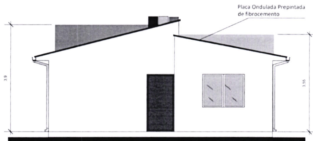
FACHADA POSTERIOR ESC.: 1:75
