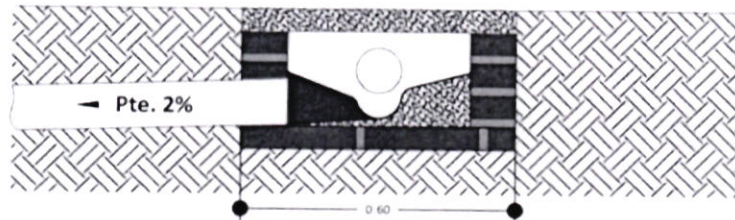
DETALLE CÁMARA DE INSPECCIÓN (0,60 x 0,60)
