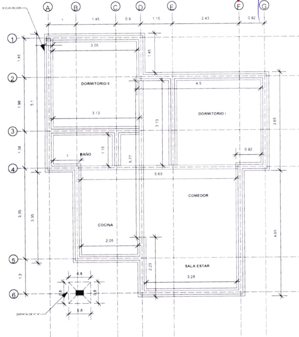
PLANO DE EXCAVACION ESC.: 1:75
