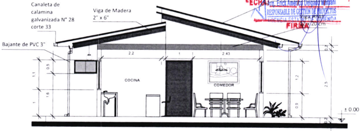
CORTE TRANSVERSAL A - A ESC.: 1:75
