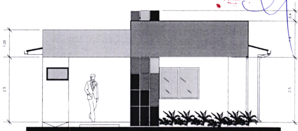
FACHADA FRONTAL ESC.: 1:75
