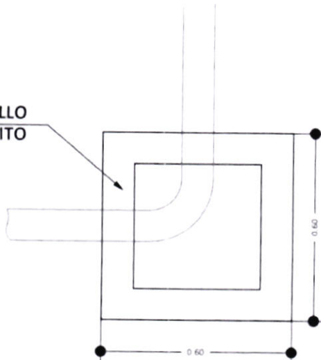
CÁMARA DE INSPECCIÓN (0,60 x 0,60)
