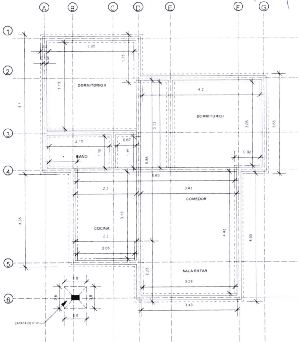
PLANO ESTRUCTURAL DE FUNDACION ESC.: 1:75
