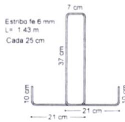
SECCION VIGA T
