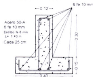
SECCION VIGA T
