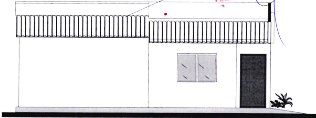
FACHADA LATERAL DERECHO ESC.: 1:75
