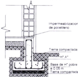
SECCIÓN ESTRIBO
