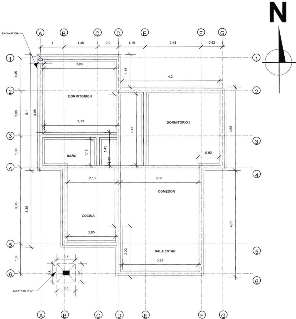
PLANO DE EXCAVACION ESC.: 1:75
