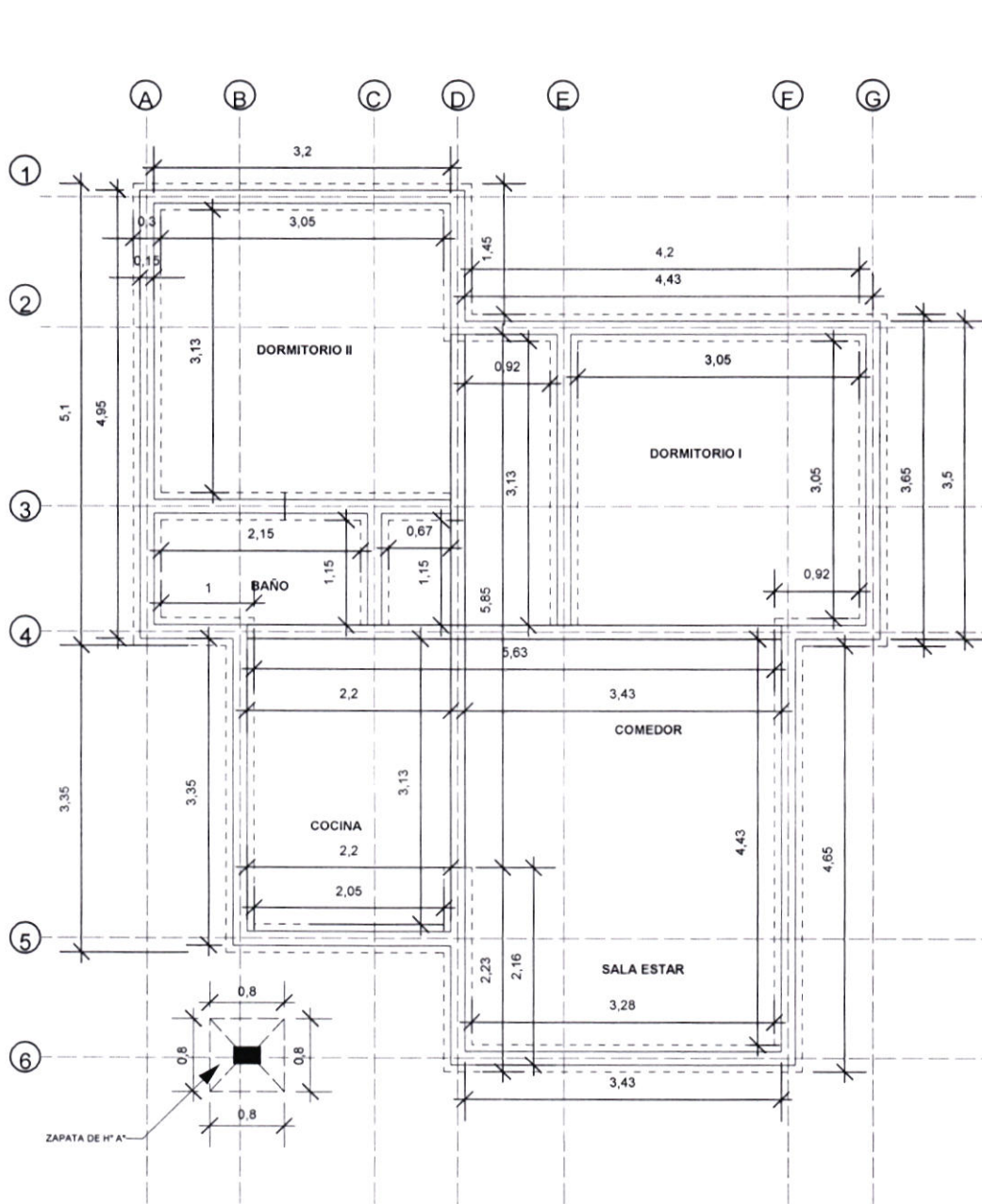
PLANO ESTRUCTURAL DE FUNDACION ESC.: 1:75
