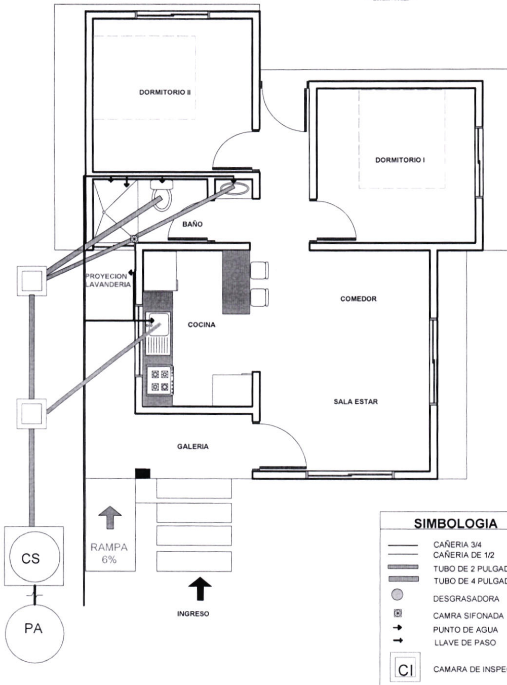
PLANO DE HIDROSANITARIO ESC.: 1:75
