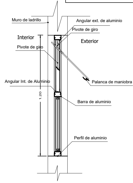
SECCION A-A
