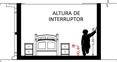
CORTE REFERENCIAL
