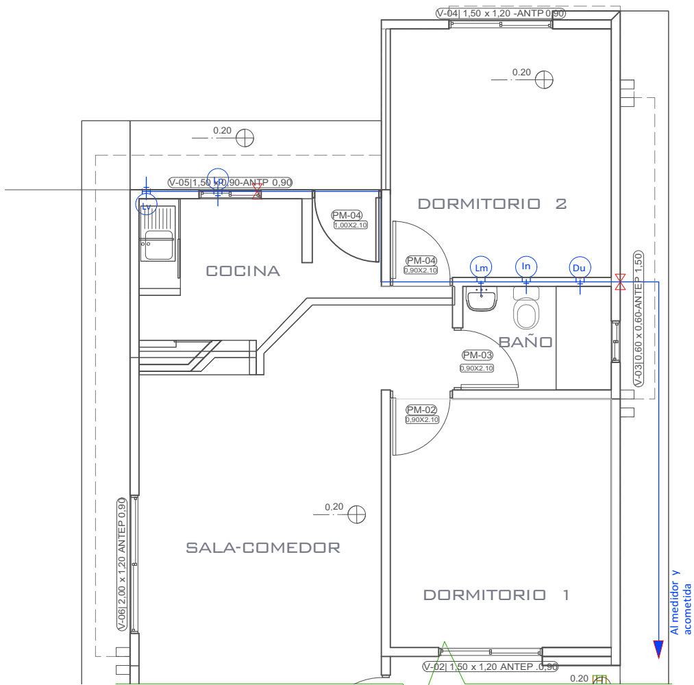
INSTALACION HIDRAULICA ESC. 1:75
