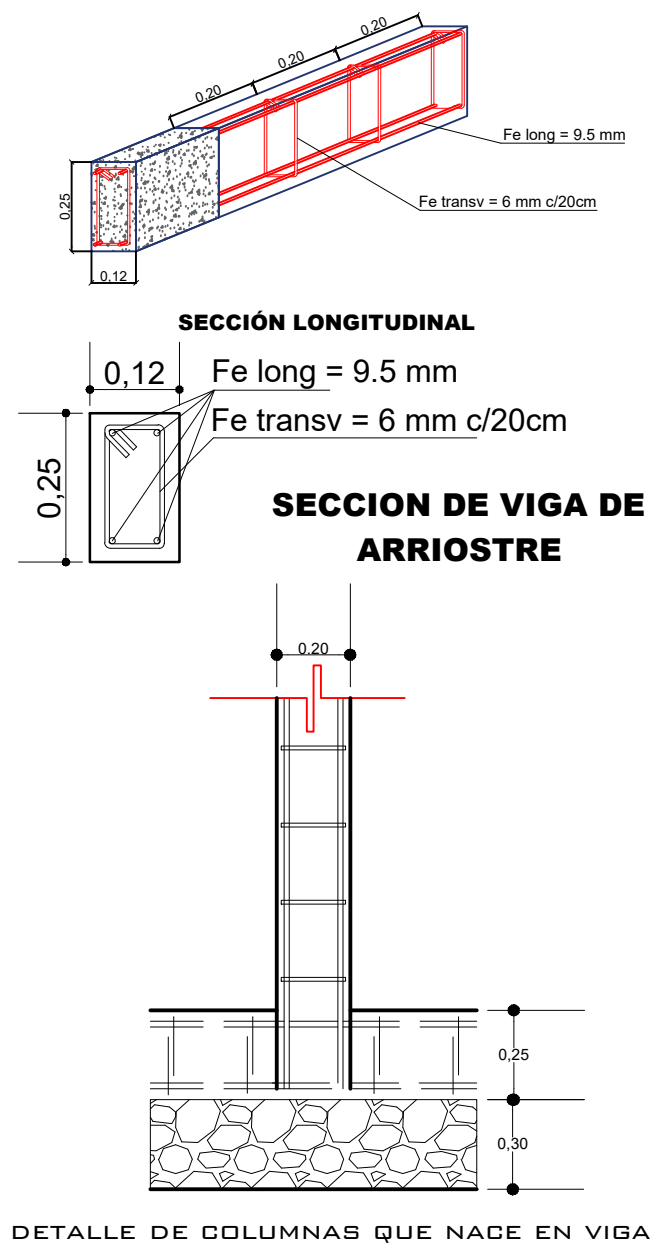
PLANO DE COLUMNAS Y VIGA ARRIOSTRE ESCALA: 1:75
