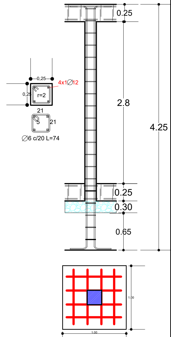
DETALLE DE COLUMNA DE TANQUE ELEVADO
