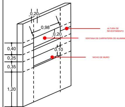
MURO DE BAÑO
