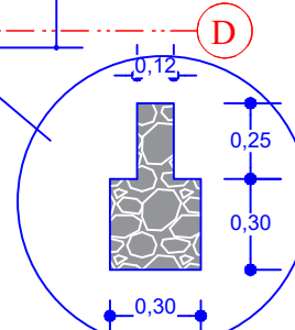
DETALLE DE CIMIENTO MURO BAÑO C 2-3
