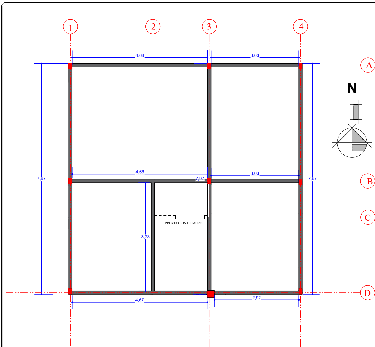
PLANO DE COLUMNAS Y VIGA ARRIOSTRE ESCALA: 1:75
