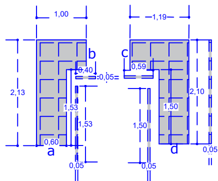
MESON DE COCINA ENCIMERA DE LAVANDERIA
