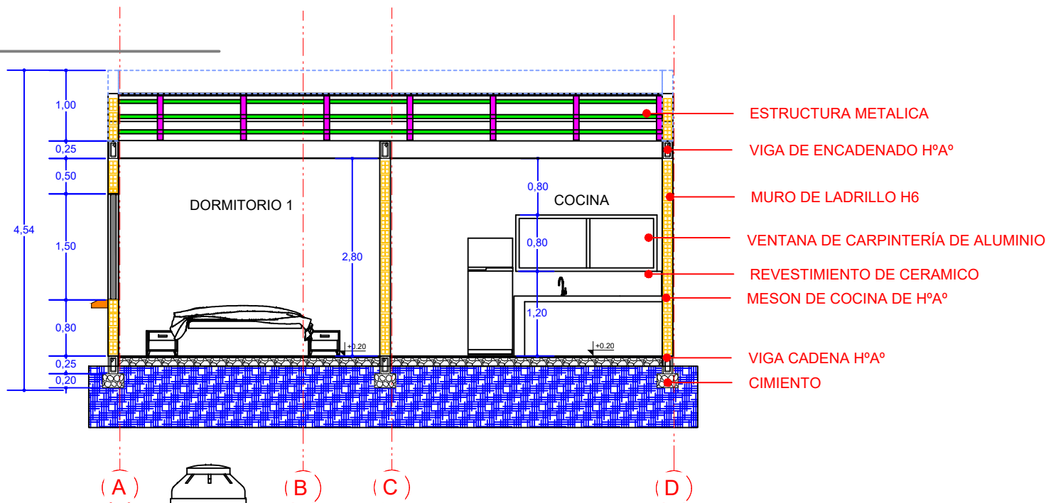
CORTE B-B
