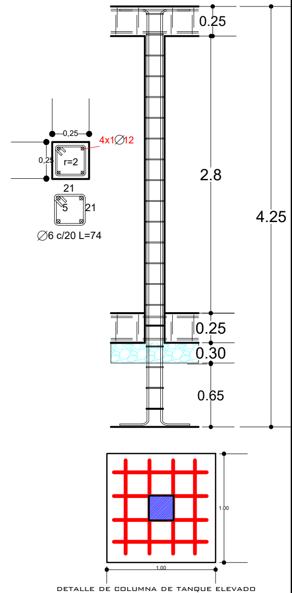
DETALLE DE COLUMNA DE TANQUE ELEVADO
