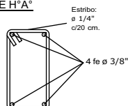
DETALLE VIGA DE Hº Aº
