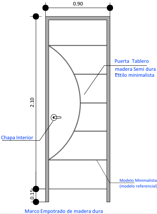
Marco Empotrado de madera dura
