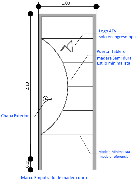
Marco Empotrado de madera dura
