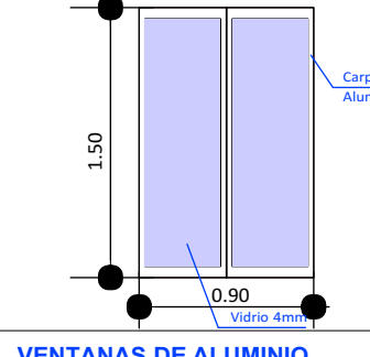
VENTANAS DE ALUMINIO LINEA 20 CON VIDRIO 4 mm
