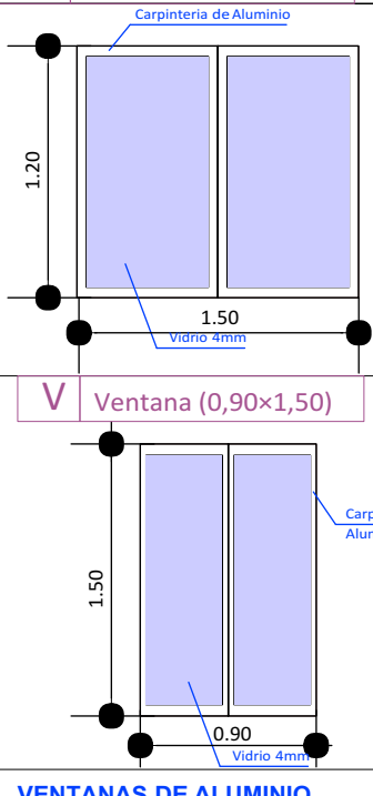
VENTANAS DE ALUMINIO LINEA 20 CON VIDRIO 4 mm
