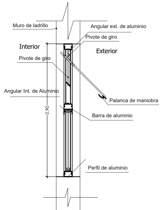
SECCION A-A
