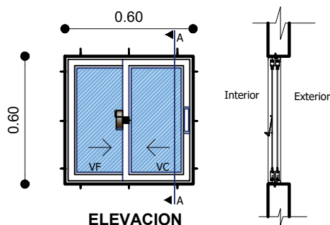
SECCION A-A
